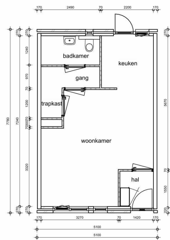
begane grond
