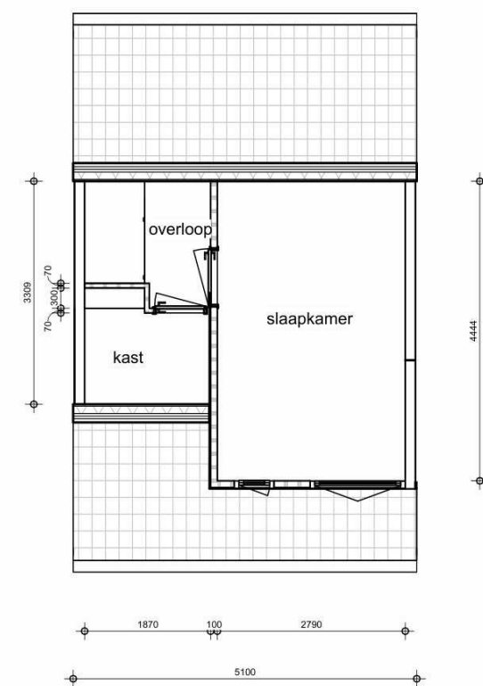
eerste verdieping
