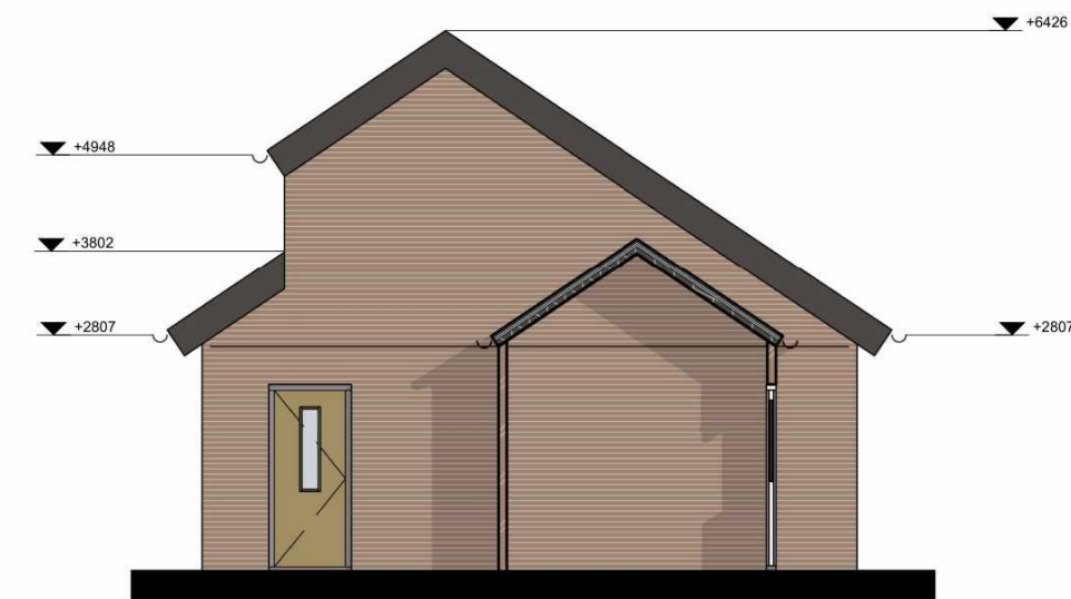
Zijgevel rechts
