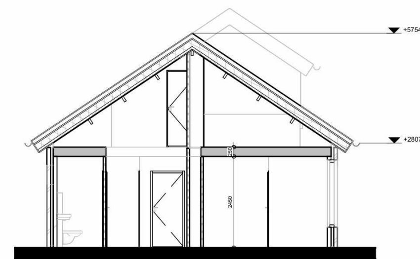
A-A
