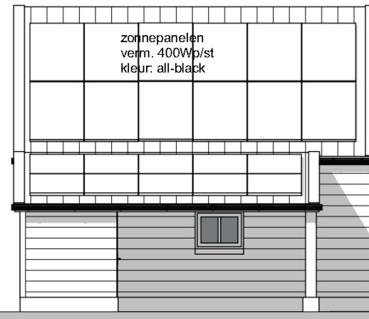
Linkergevel bijgebouw
