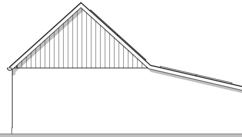
Achtergevel Bijgebouw
