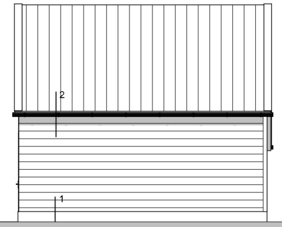
Rechtergevel bijgebouw
