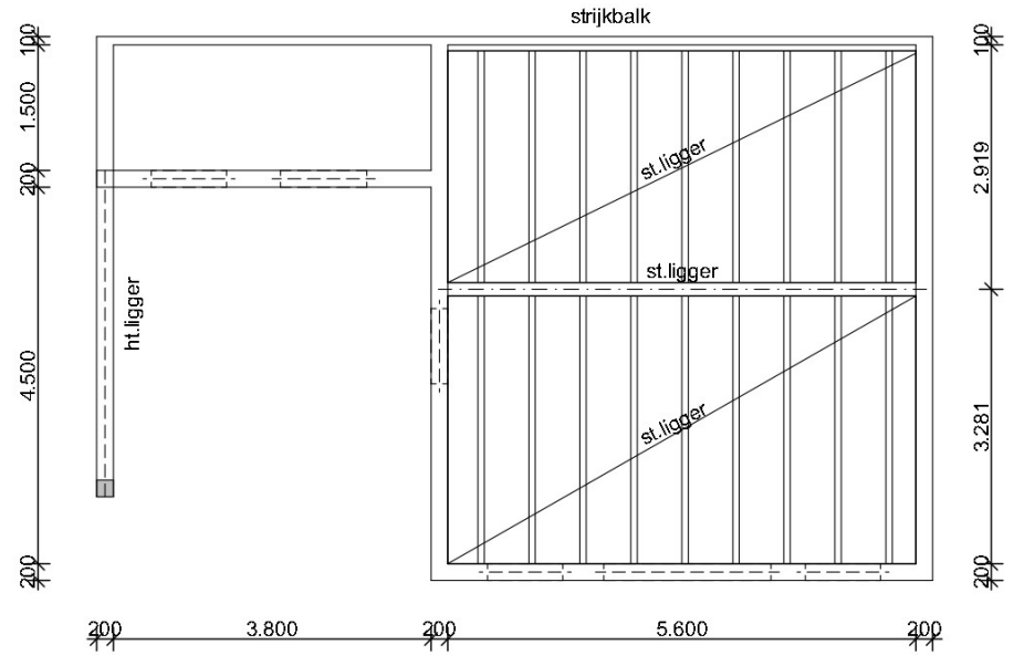
Balklagen
