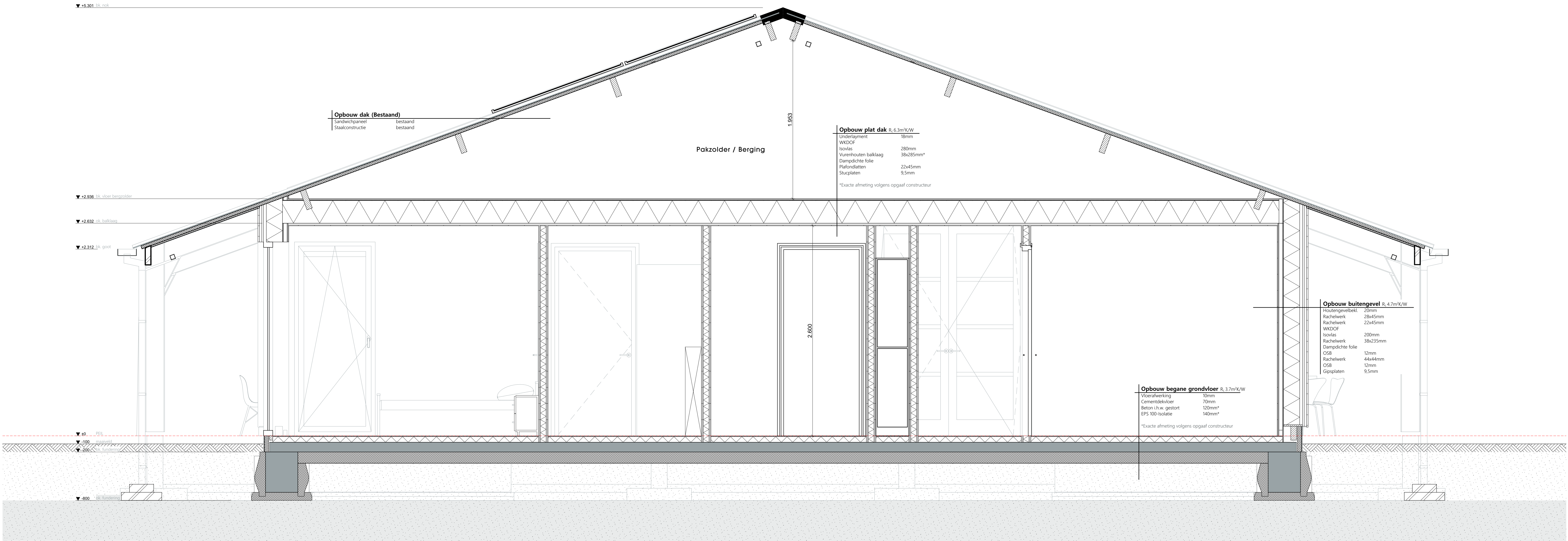
Principe doorsnede A-A
