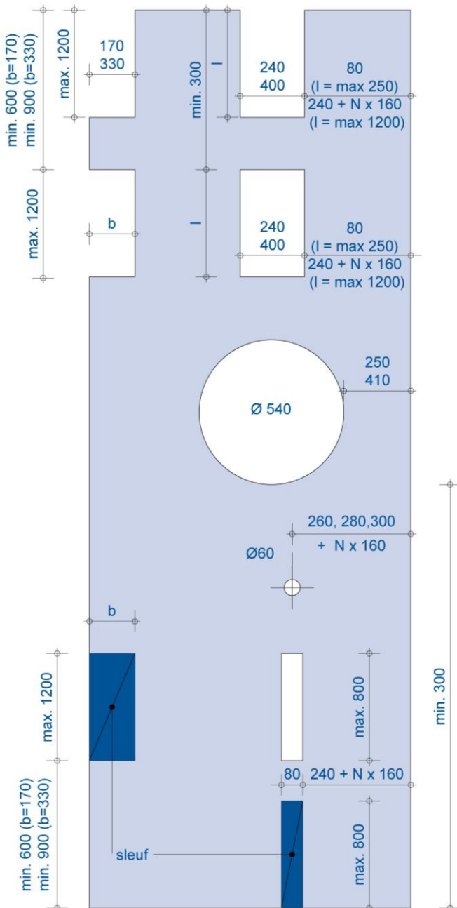
Mogelijkheden voor het fabrieksmatig aanbrengen van sparingsen
