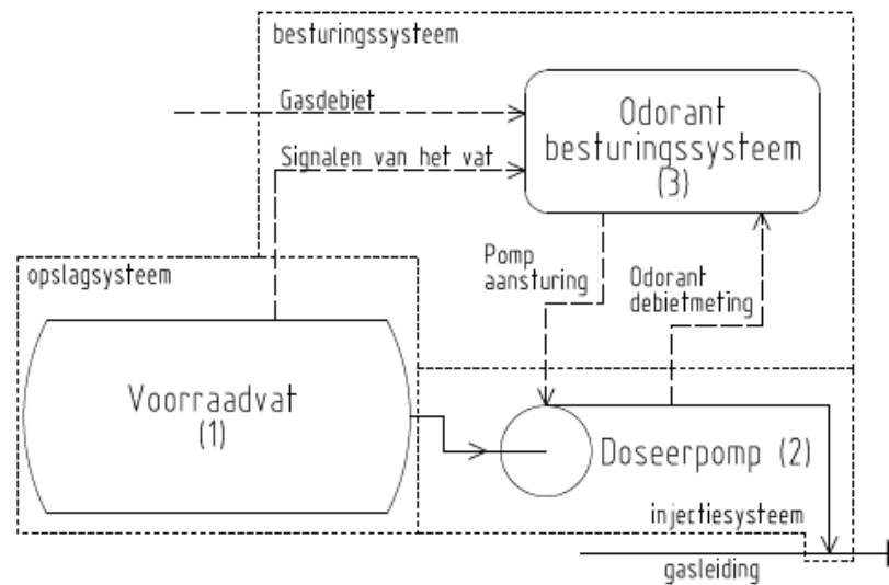
Figuur 2 – Schematische weergave odorantsysteem
