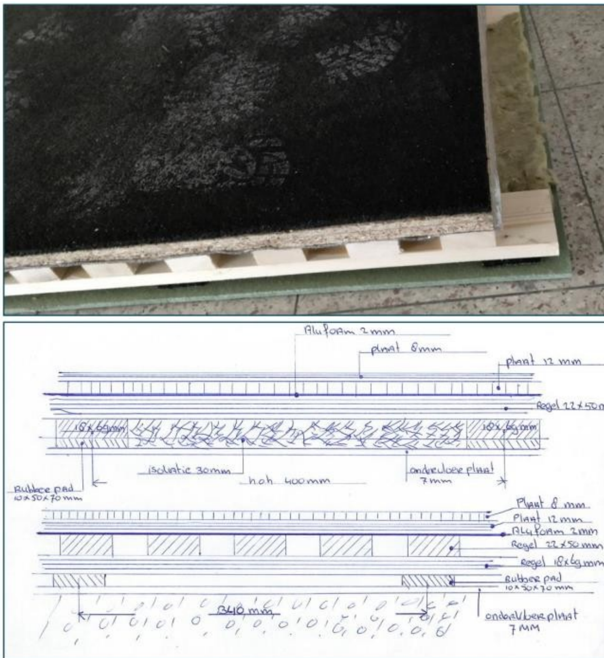
Figuur 3 Principe opbouw houten zwevende sportvloer
