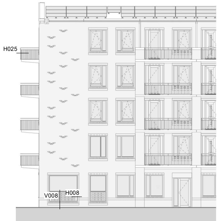
blok B2 Voorgevel Noord
