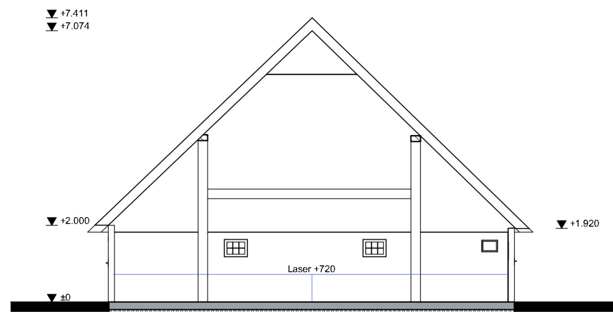
Doorsnede A-A
