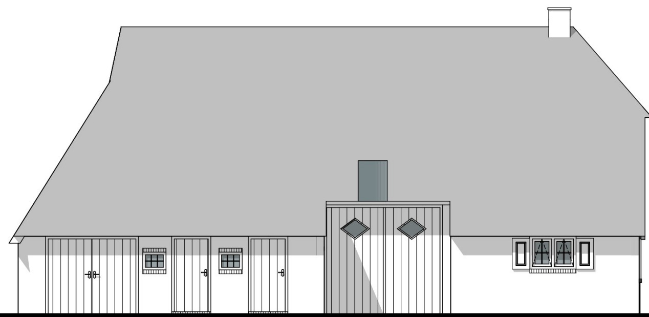
Linkergevel
