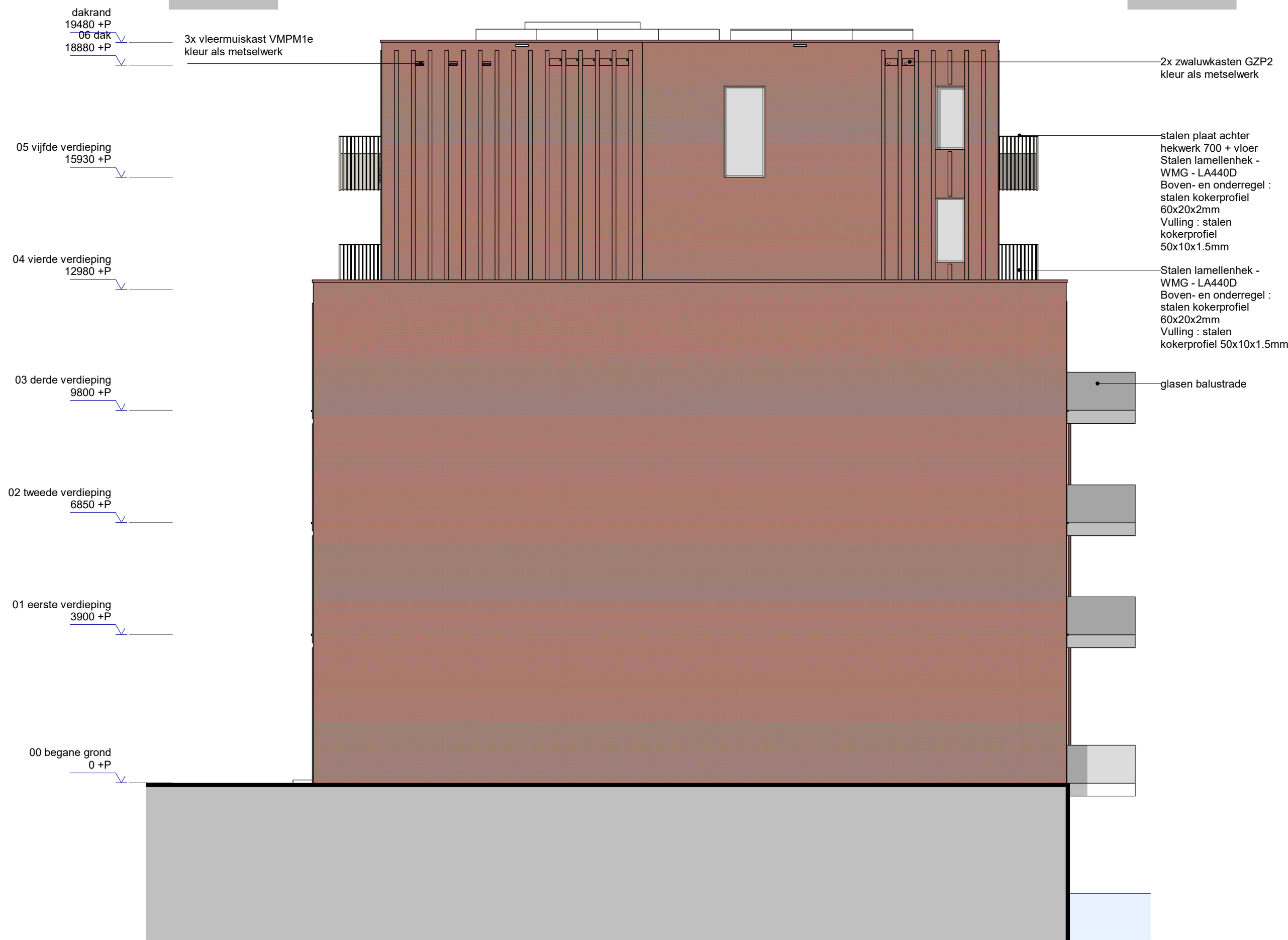
oostgevel
