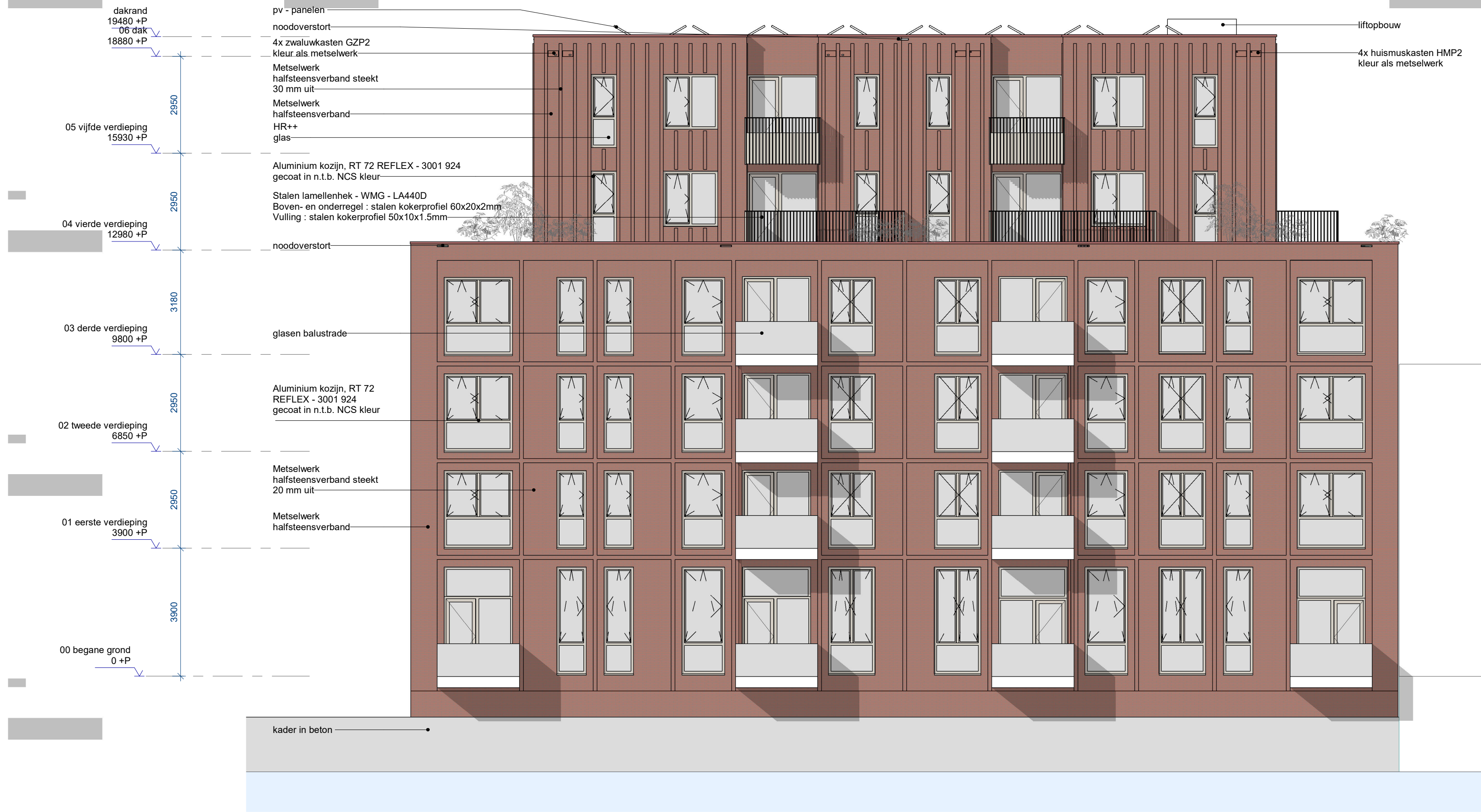
noordgevel
