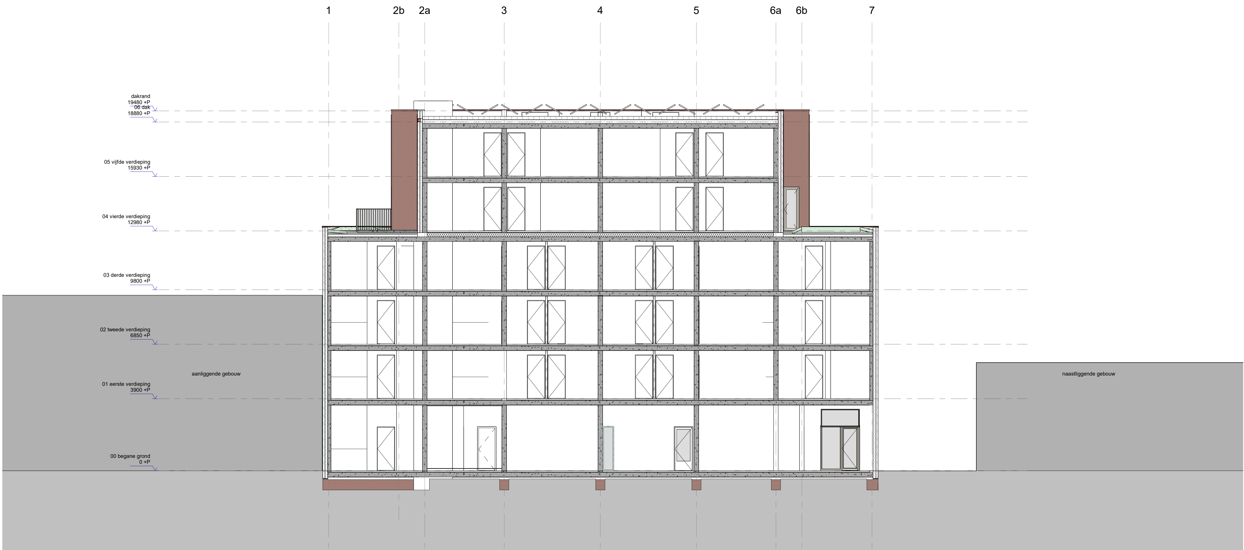
doorsnede B
