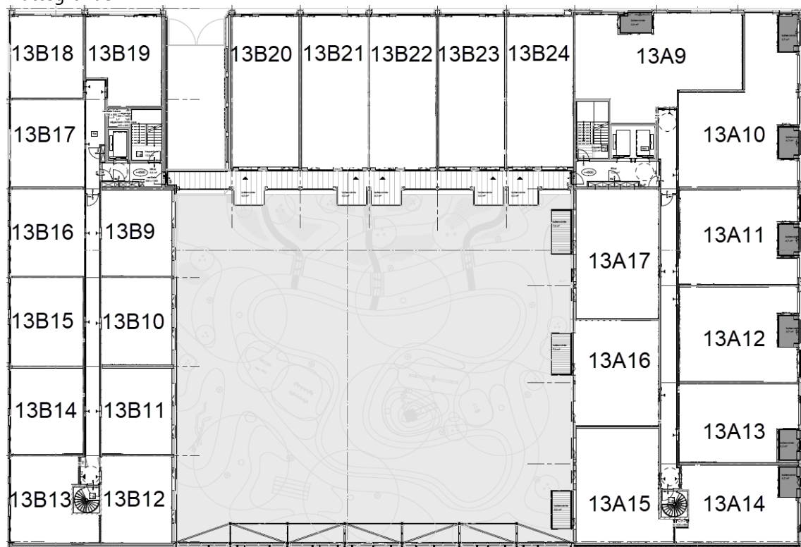
Verdieping 1
