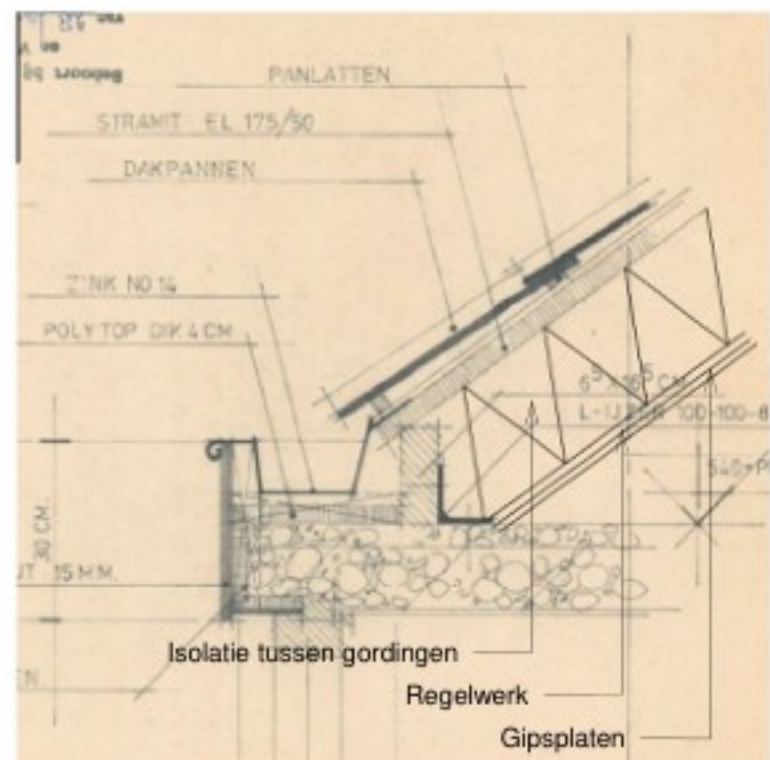
Detail dakopbouw nieuw 1 : 20
