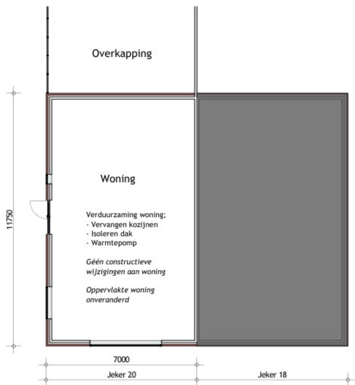
Begane grond 1 : 100
