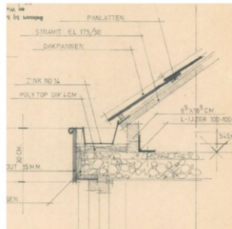
Detail dakopbouw bestaand 1 : 20
