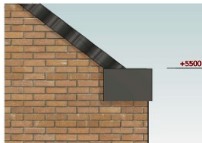
Aanzicht goot bestaand/nieuw 1 : 20
