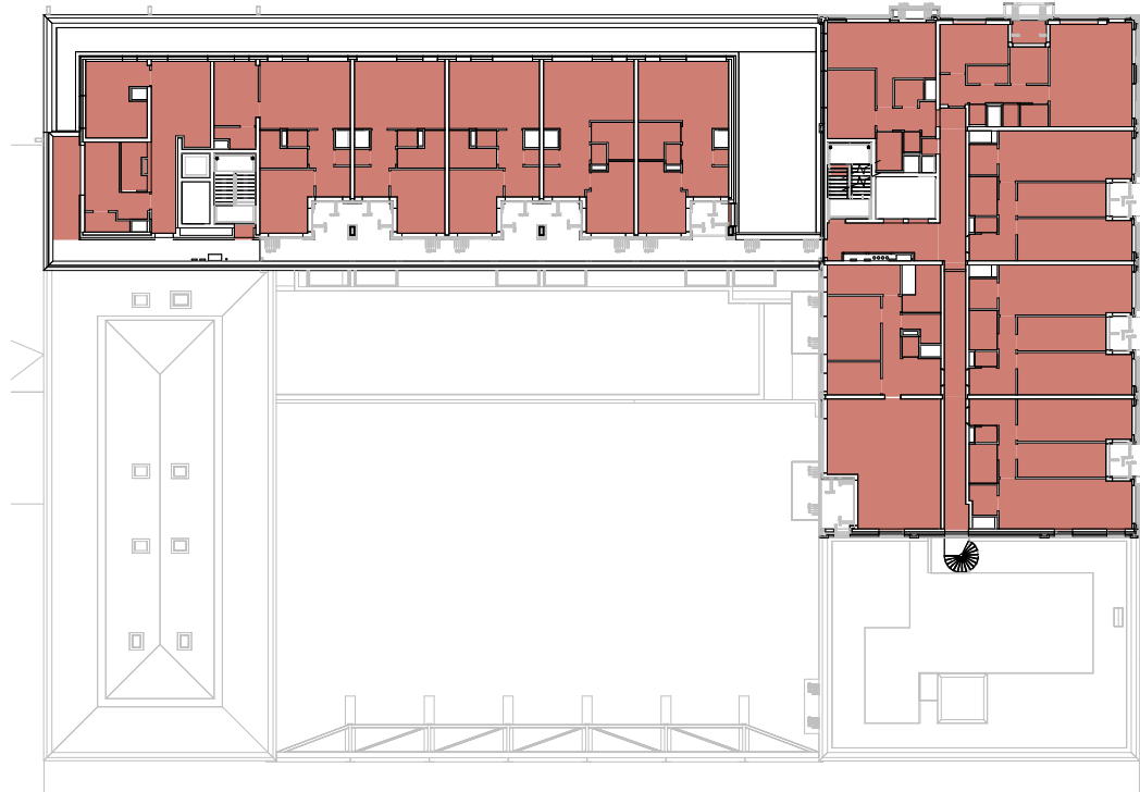
07 zevende verdieping
