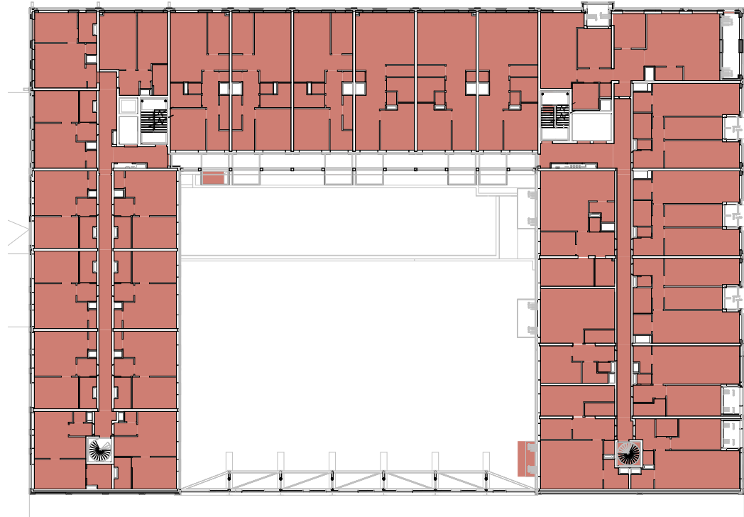
04 vierde verdieping
