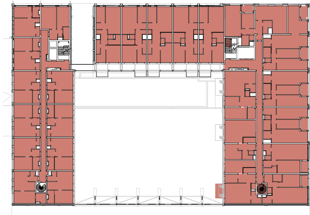
01 eerste verdieping
