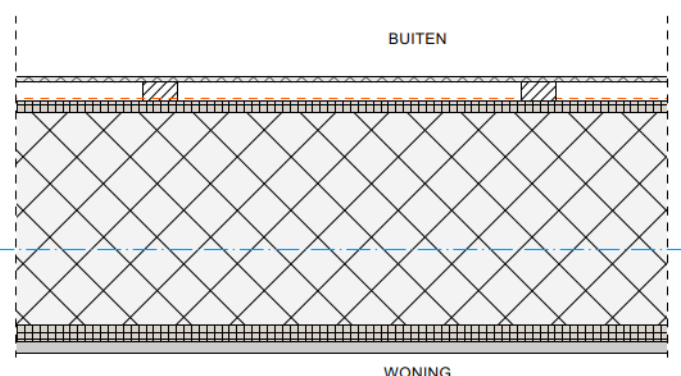
Detail gevelelement
