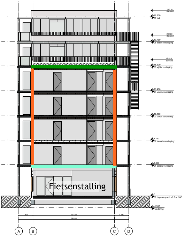
Dwarsdoorsnede F-F
