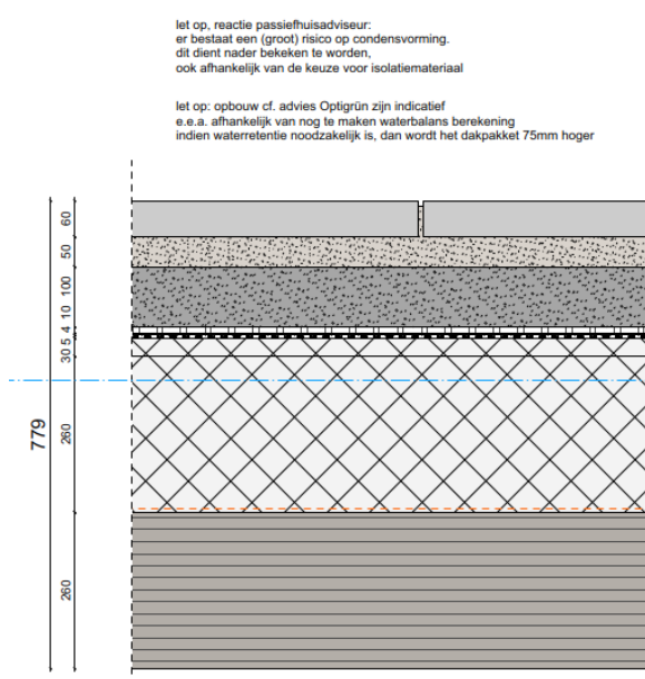
Detail opbouw vloer dakterras
