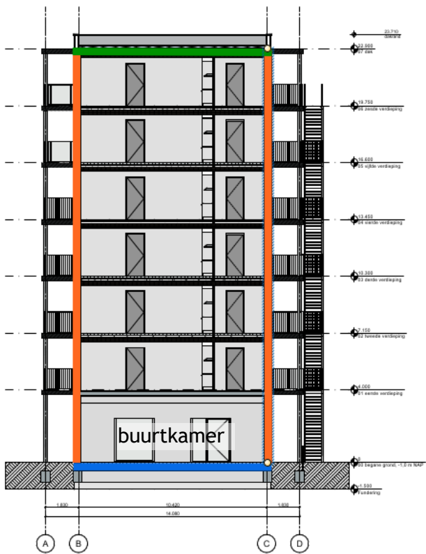
Dwarsdoorsnede A-A
