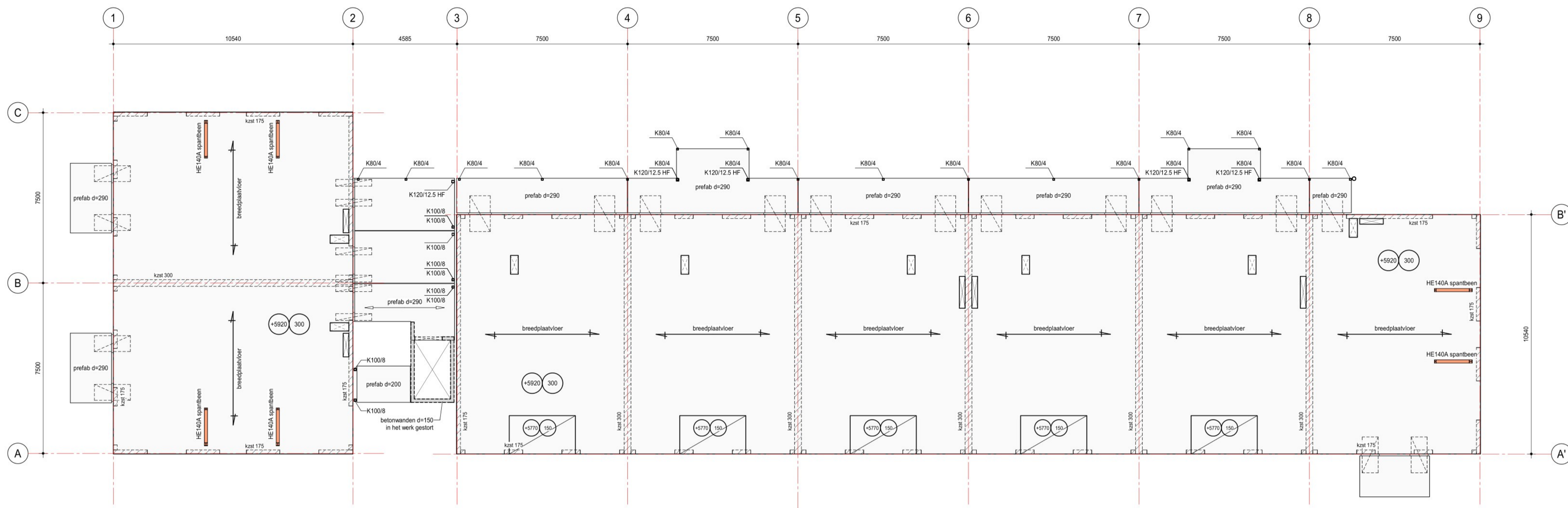
2e verdiepingvloer
