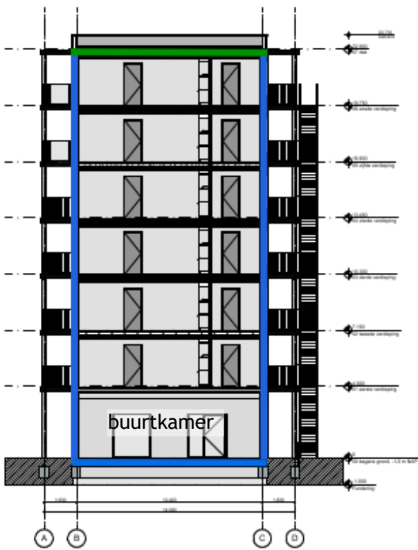
Dwarsdoorsnede A-A
