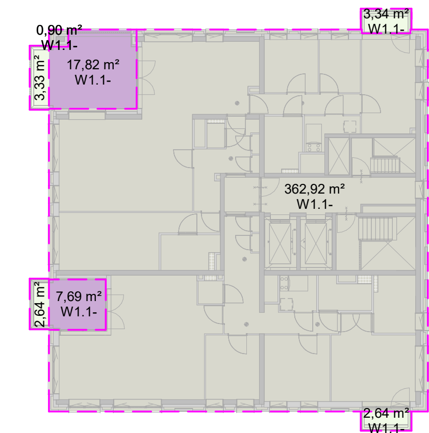
Elfde verdieping W1.1-W1.2-W1.3
