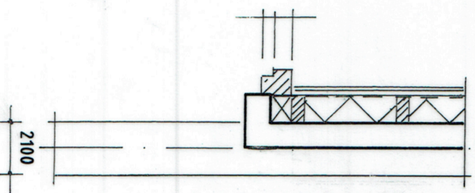
SCHAAL DETAILS 1 : 20.
