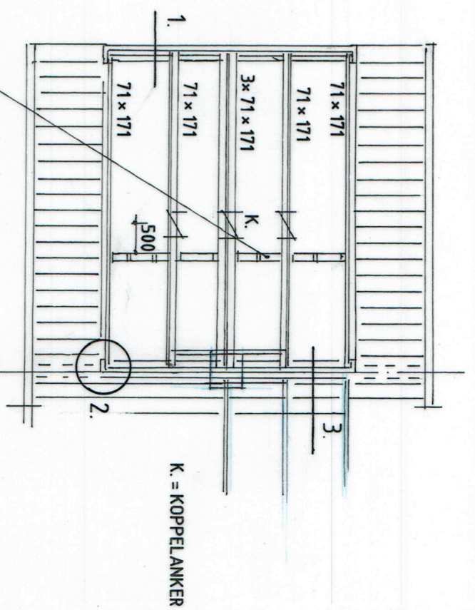
KAPPLAN GEWIJZIGD
