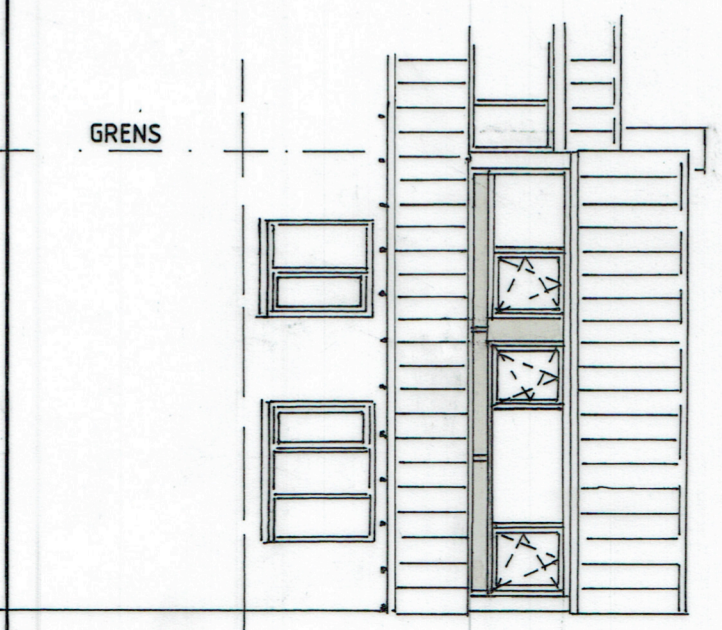
ACHTERAAANZICHT GEWIJZIGD
