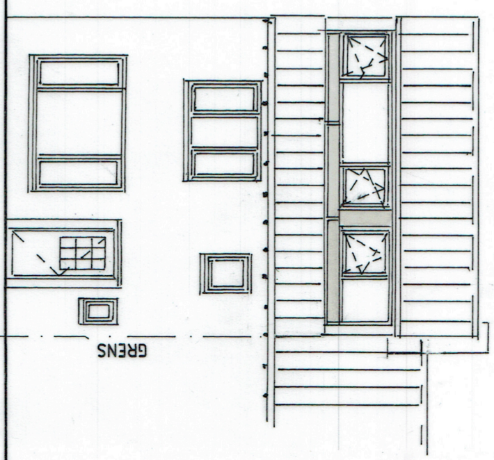
VOORAANZICHT GEWIJZIGD
