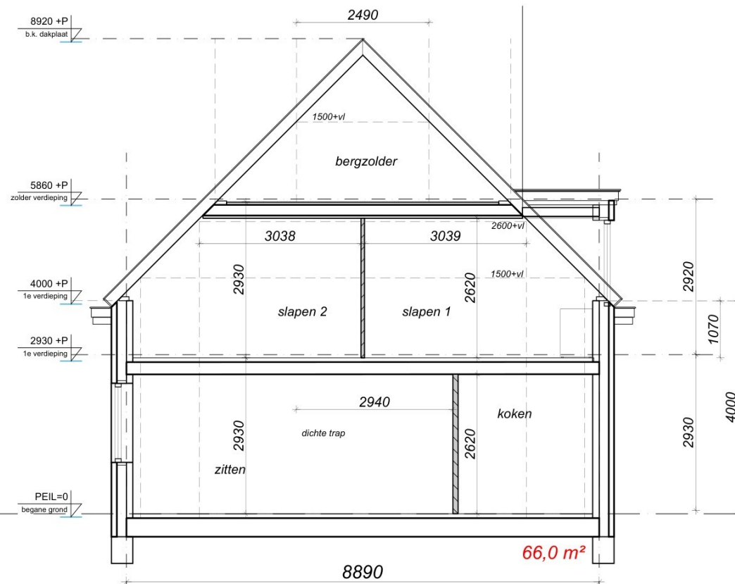
doorsnede A - A
