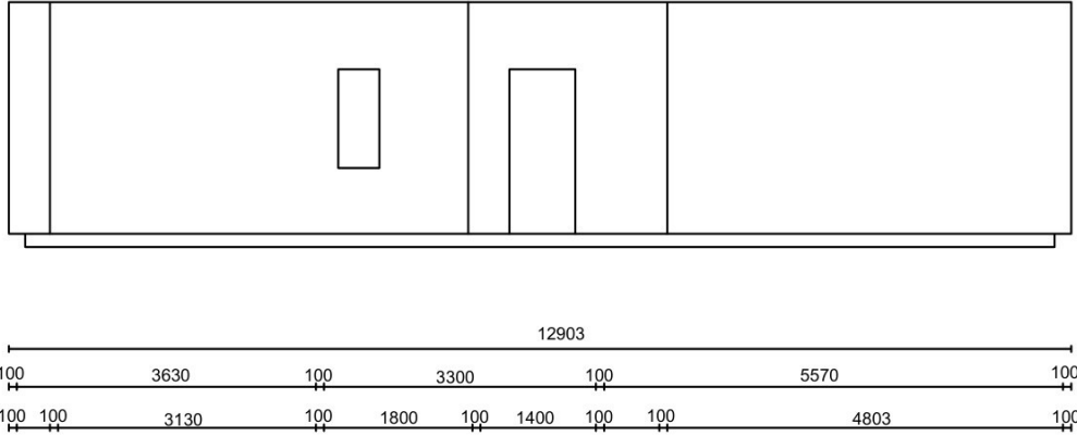
AANZICHT: D
