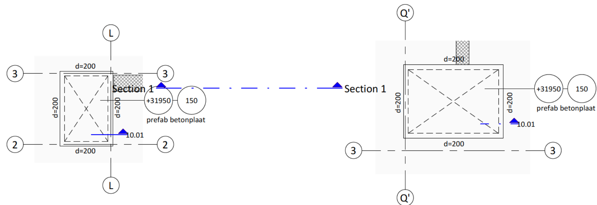
tiende verdieping - liftopbouw AS L
