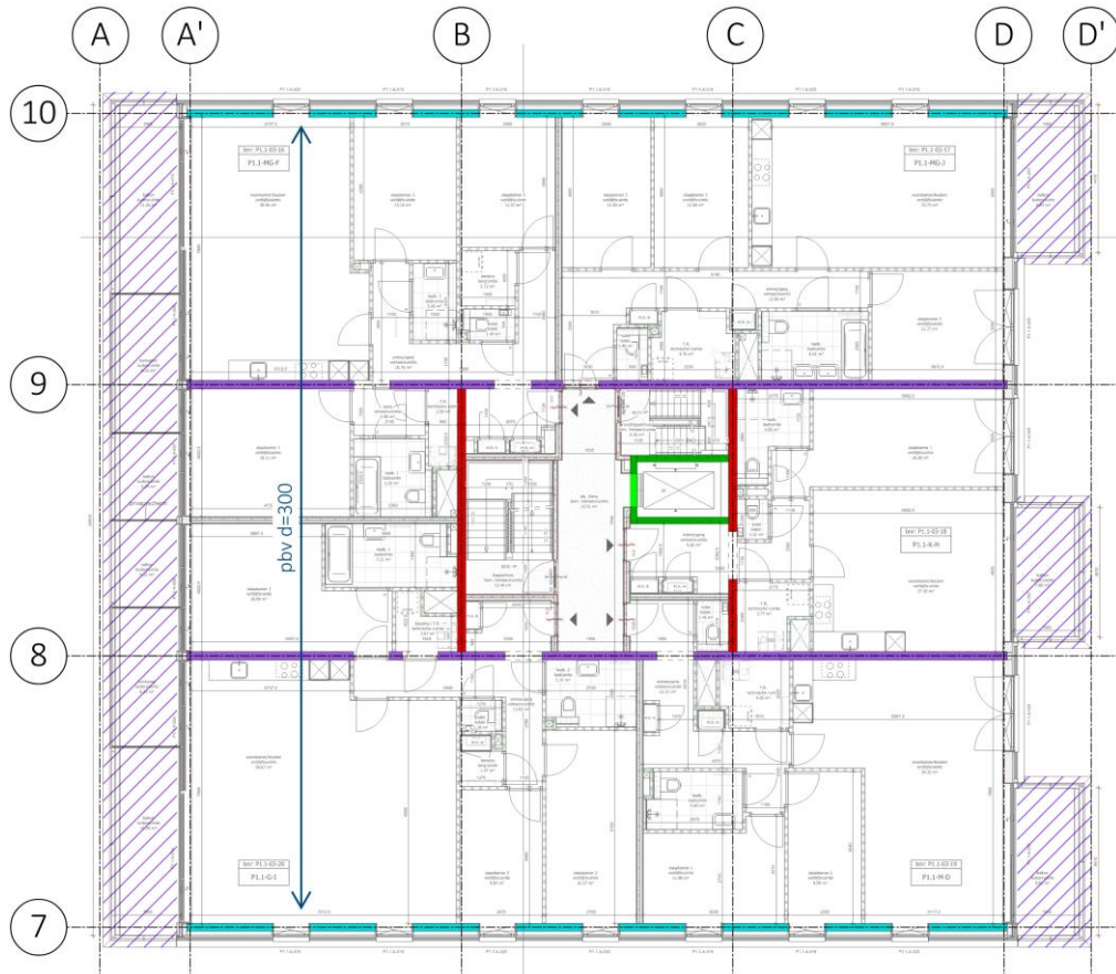
Stabiliteitsvoorzieningen evenwijdig aan letter- en cijferassen
