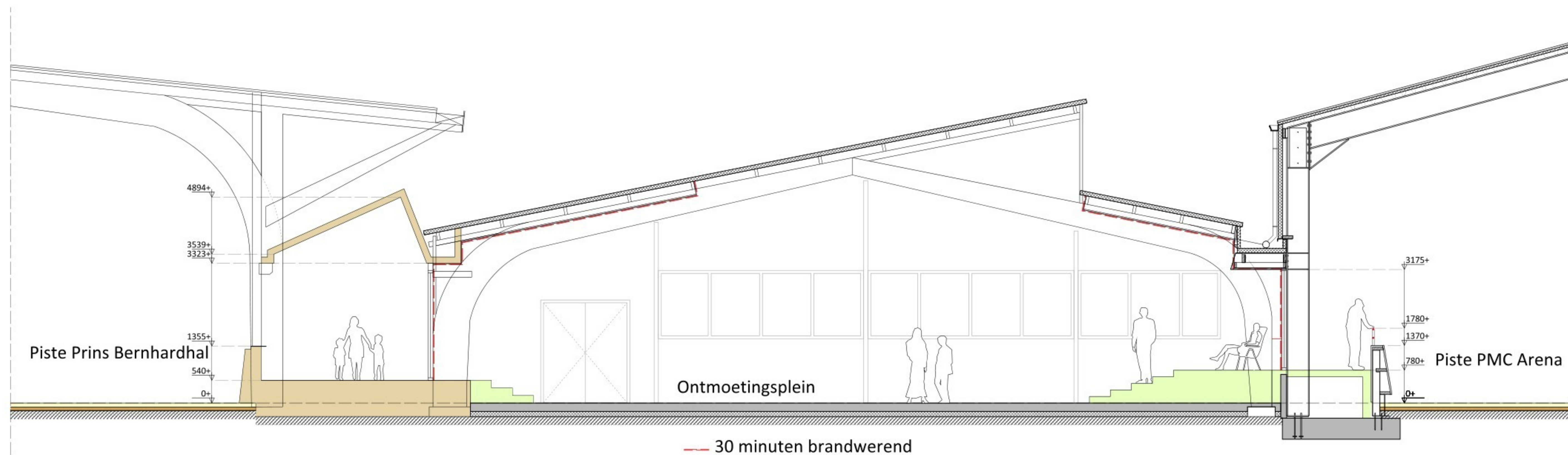
---- Doorsnede A Bestaand ----
