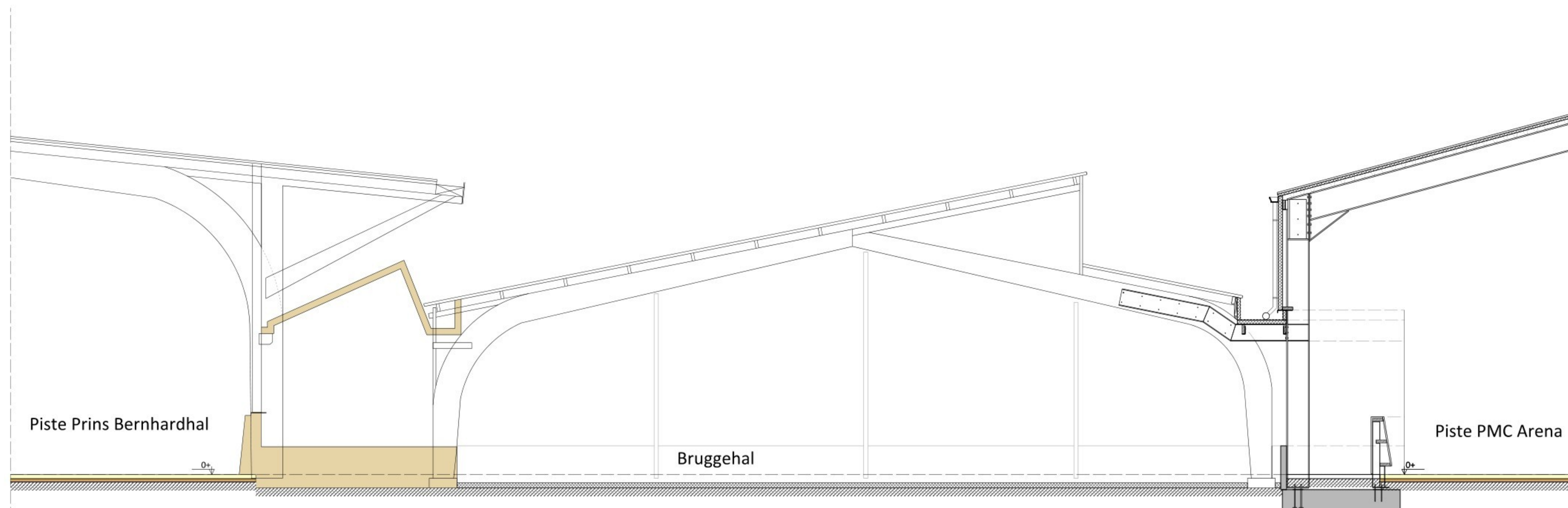
---- Doorsnede A Bestaand ----
