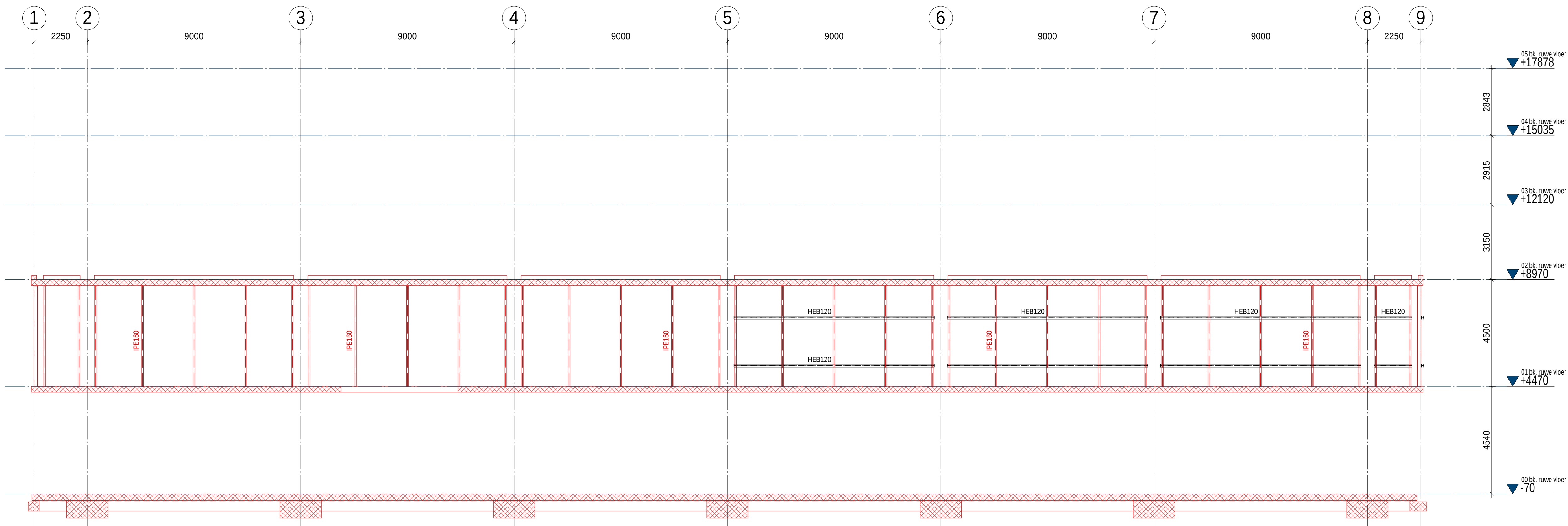
Aanzicht as F 1 : 100
