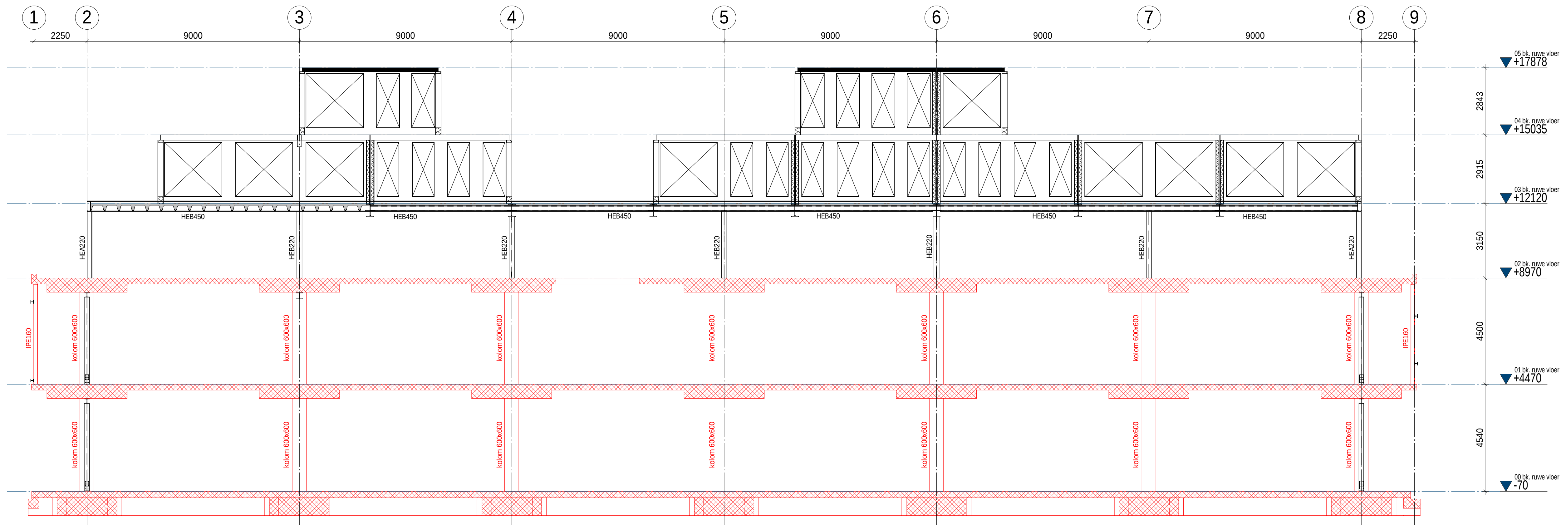
Aanzicht as E 1 : 100
