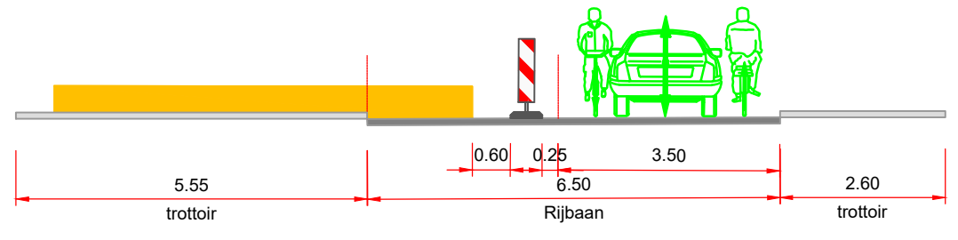
Dwarsprofiel B-B
