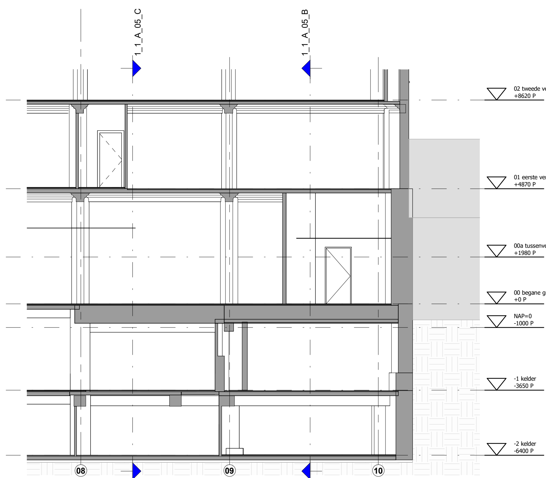
03_doorsneden_fragment 1.1_A_05_A
