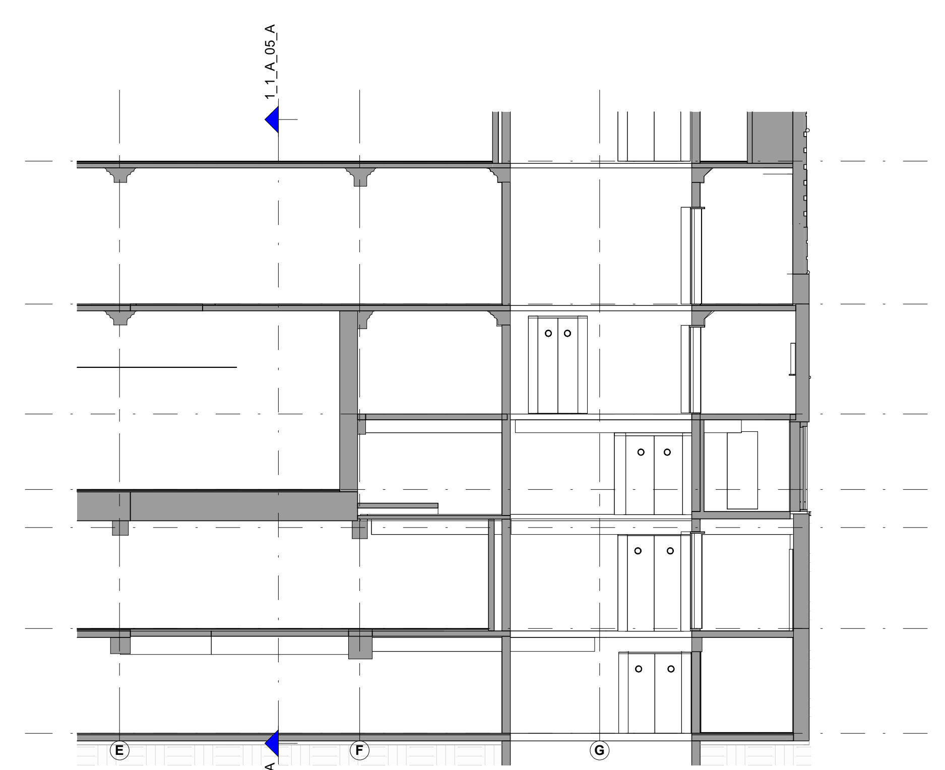
03_doorsneden_fragment 1.1_A_05_C
