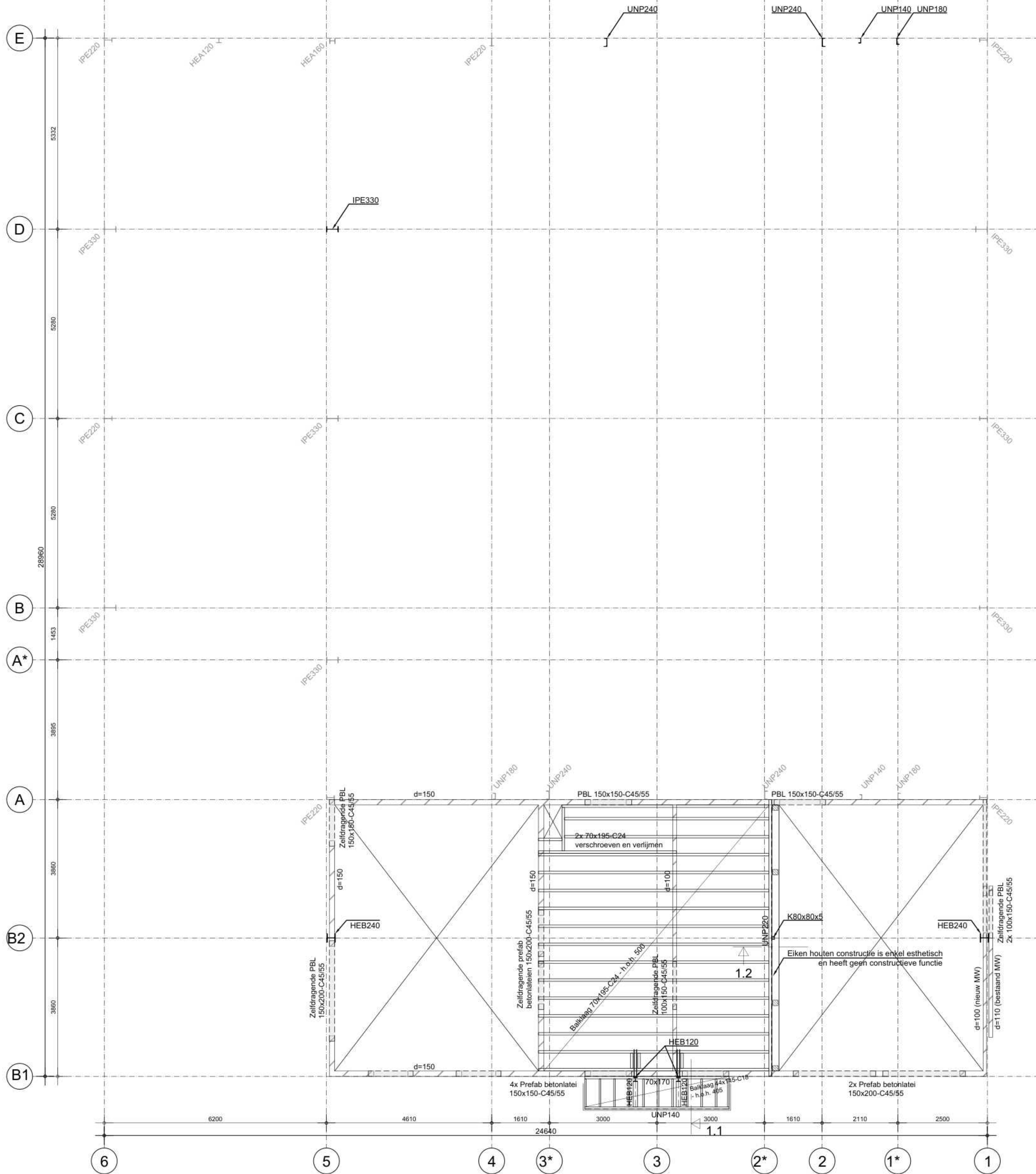
1 e verdiepingvloer praktijkruimte
