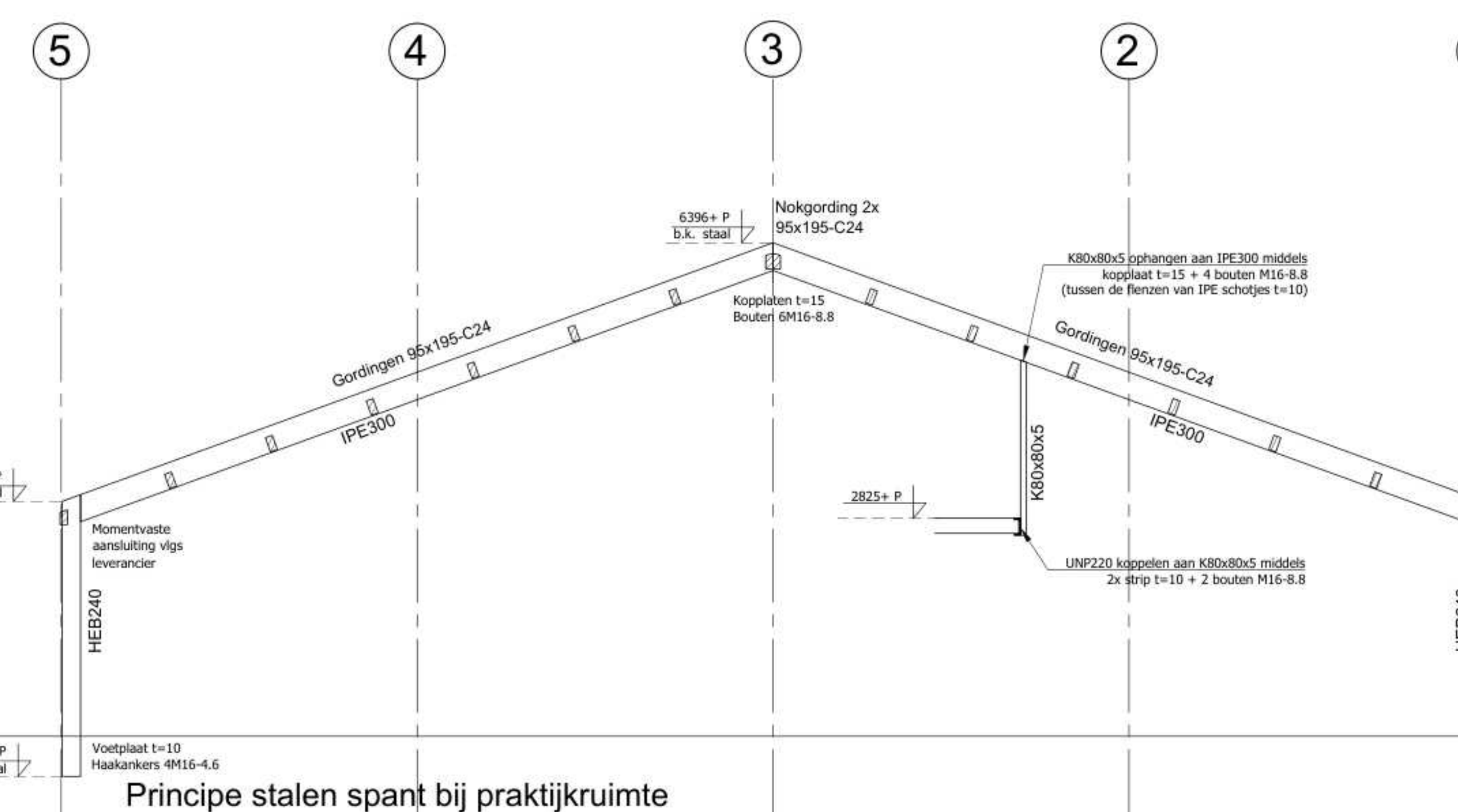
Principe stalen spant bij praktijkruimte
