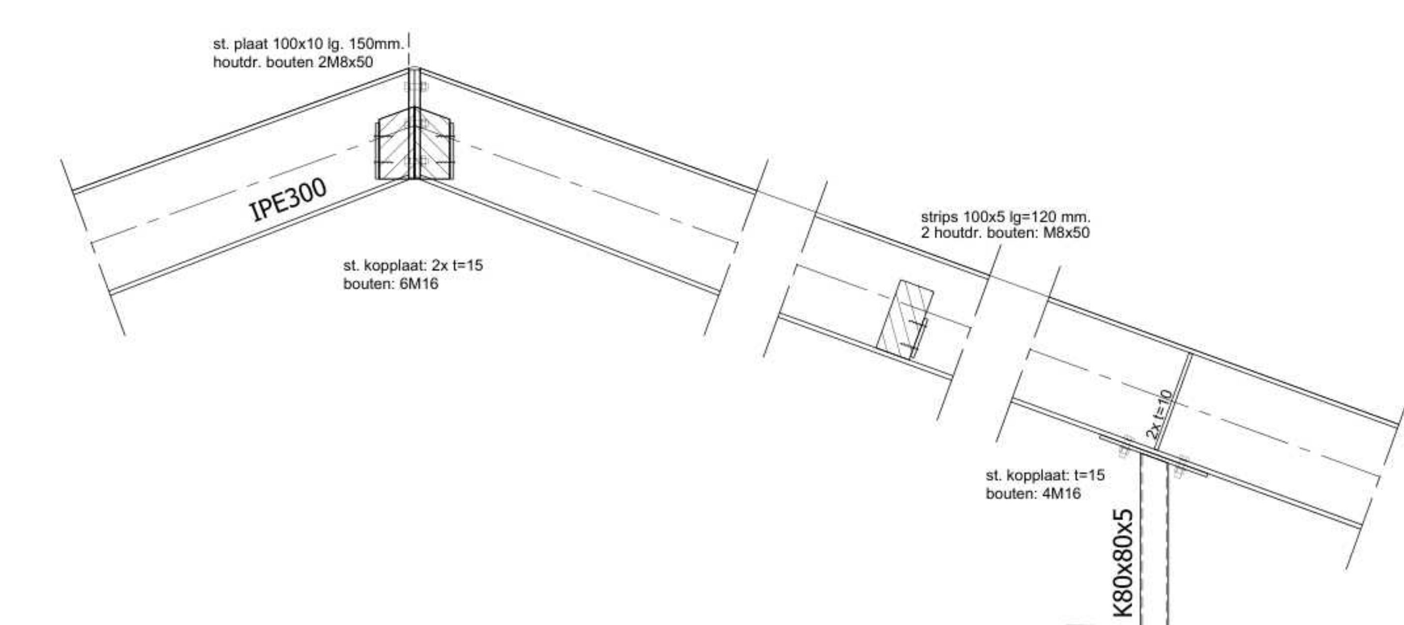
Principe stalen spant bij praktijkruimte
