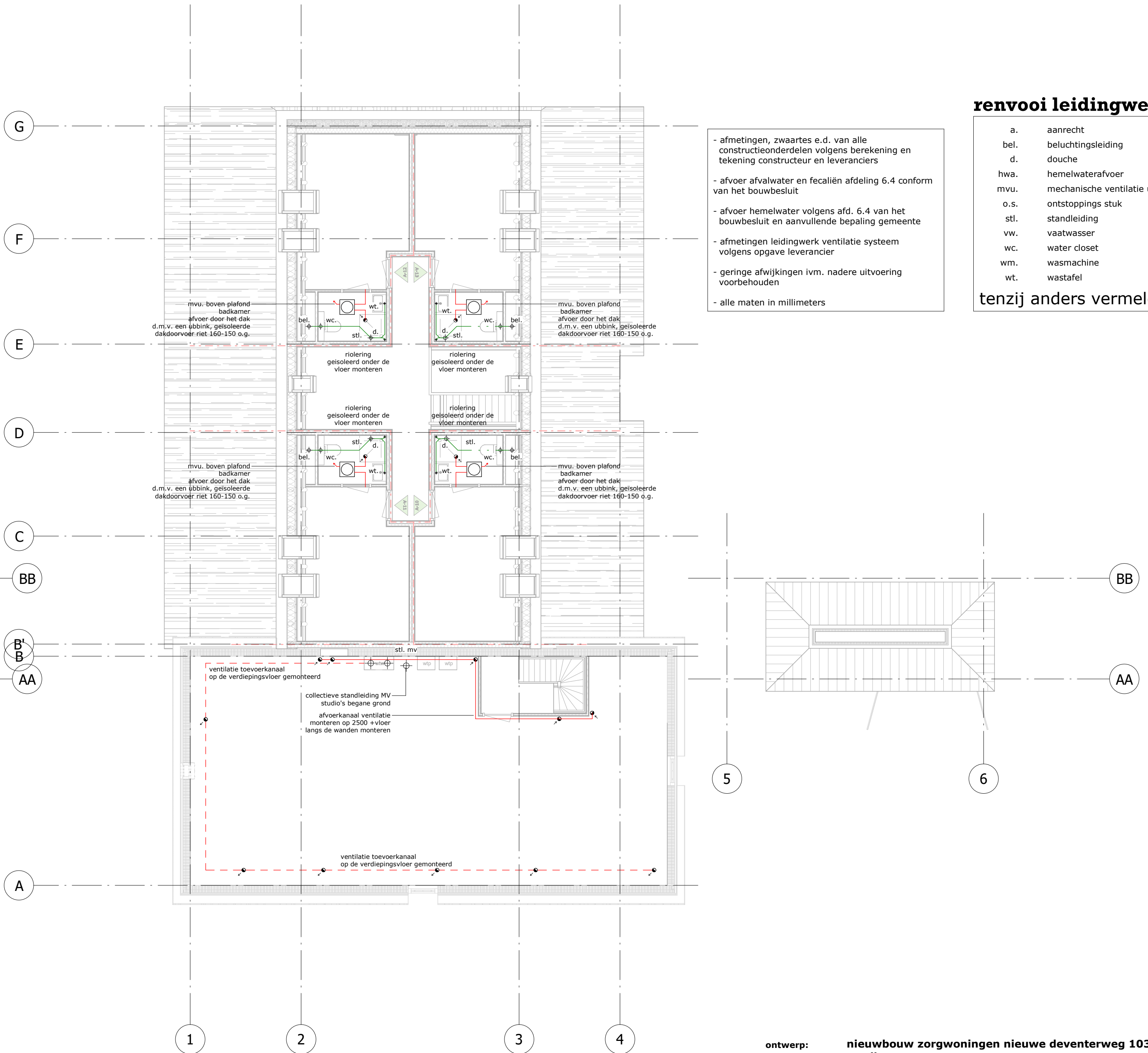
verdieping, riolering- en ventilatieplan
