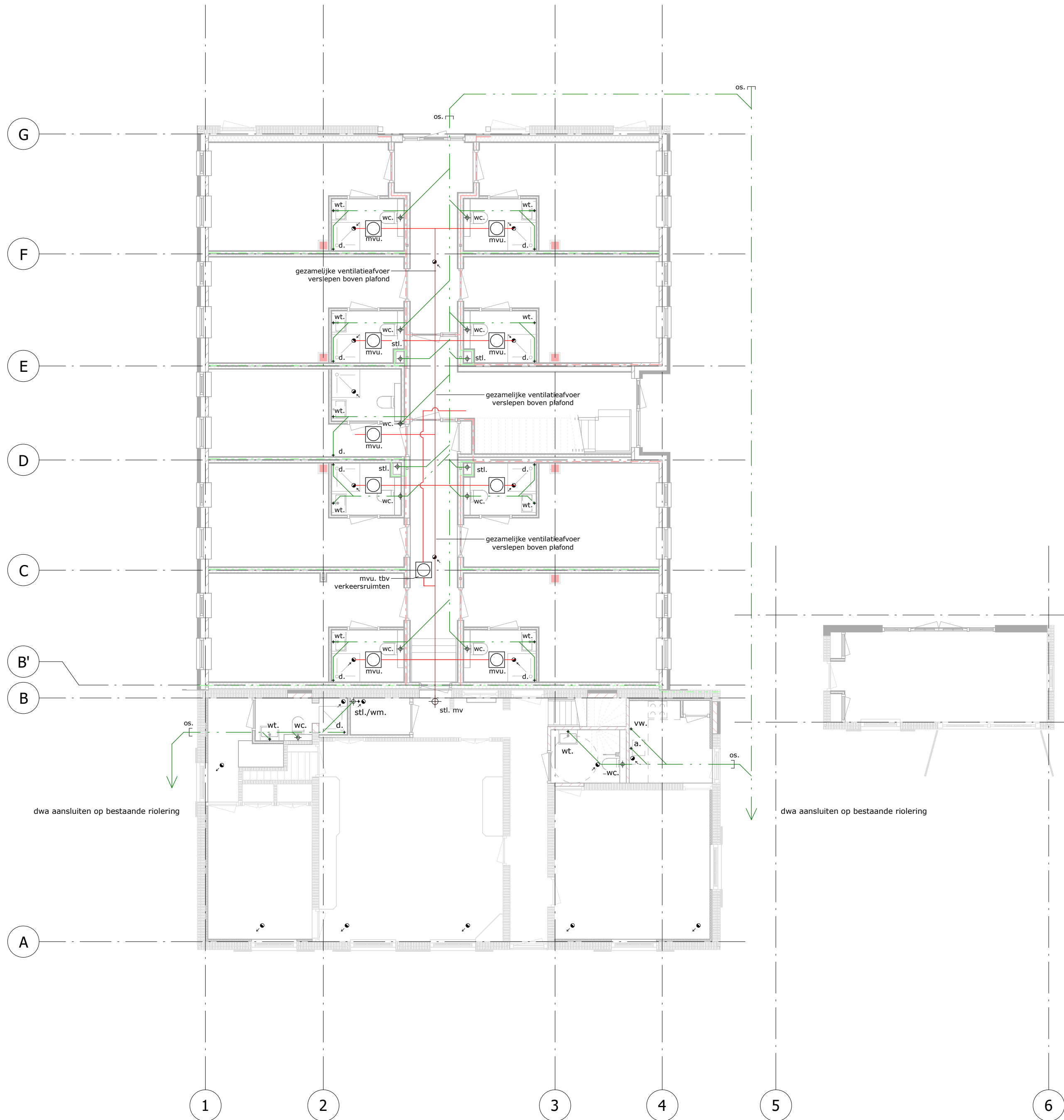
begane grond, riolering- en ventilatieplan
