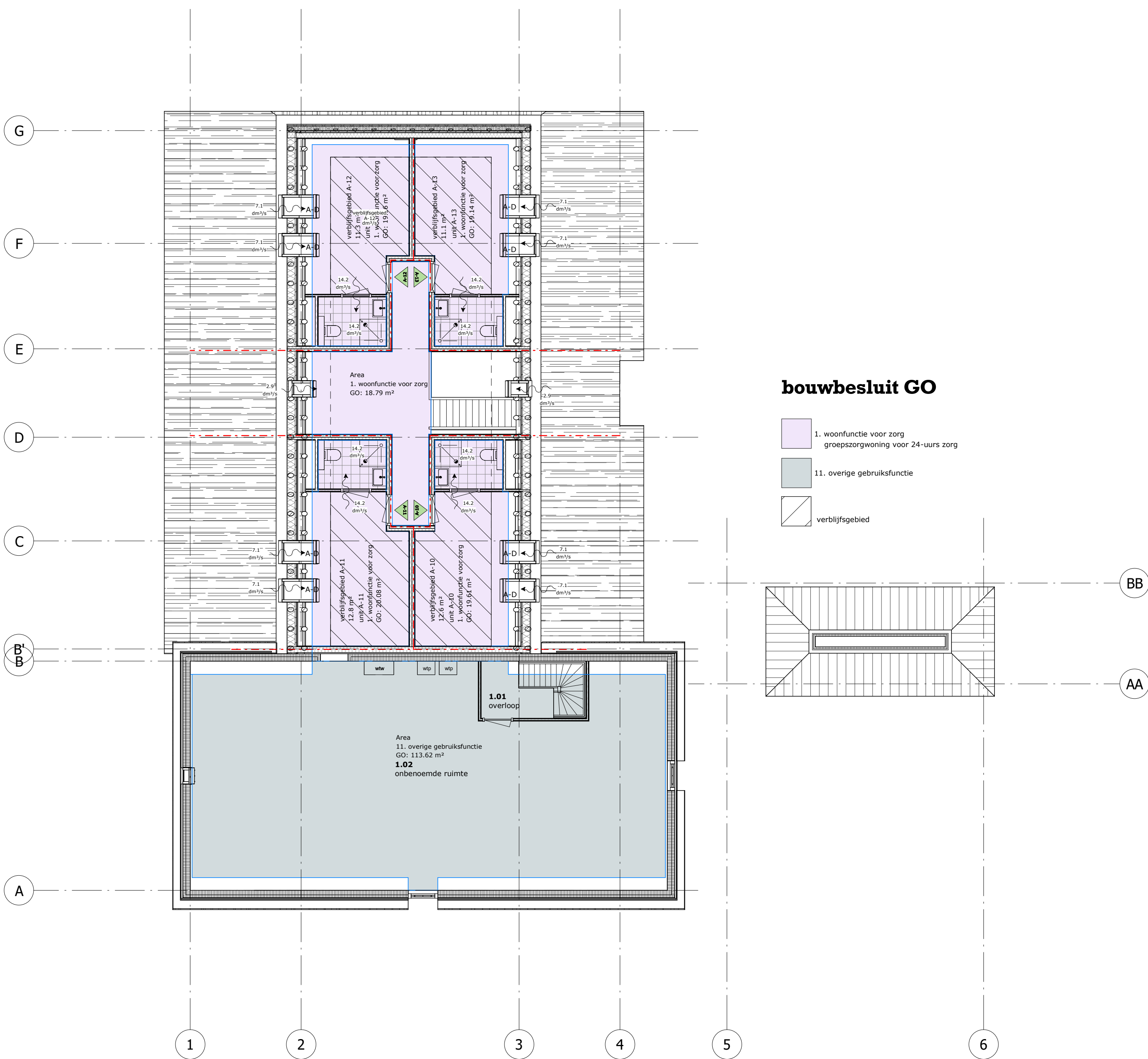
verdieping, bouwbesluit en stromingsschema
