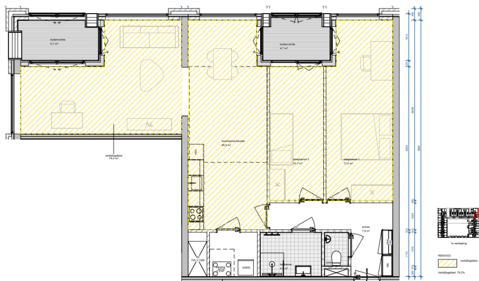
f 5.26 Woningtype C9
