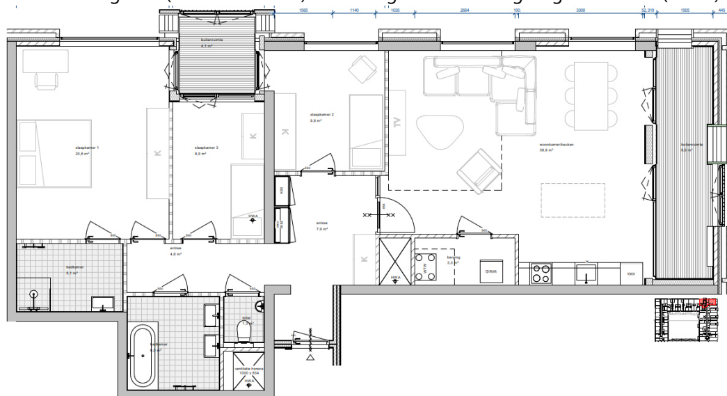
f 5.18 Woningtype C2
