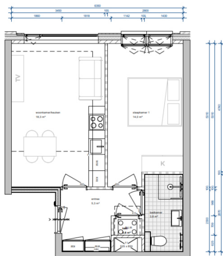
f 5.6 Woningtype B3
