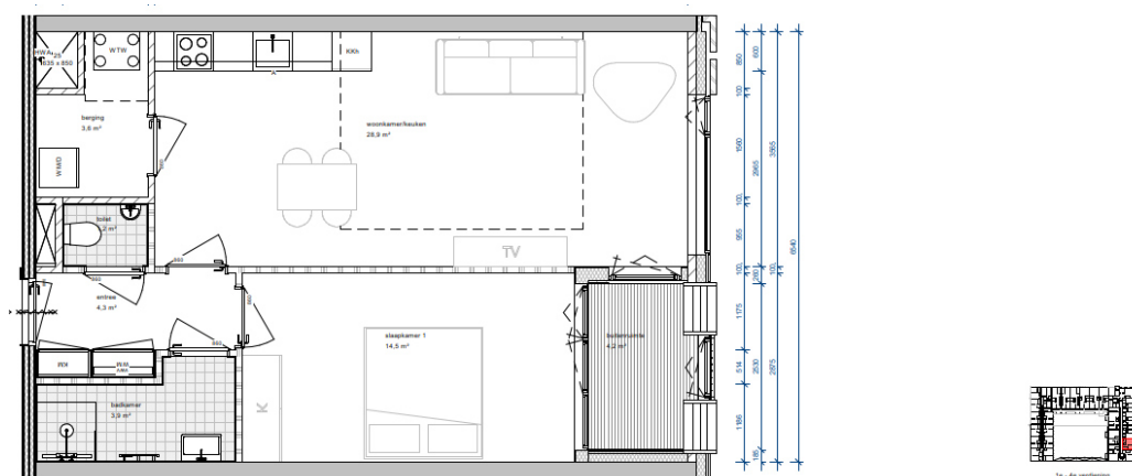
f 5.30 Woningtype D4
