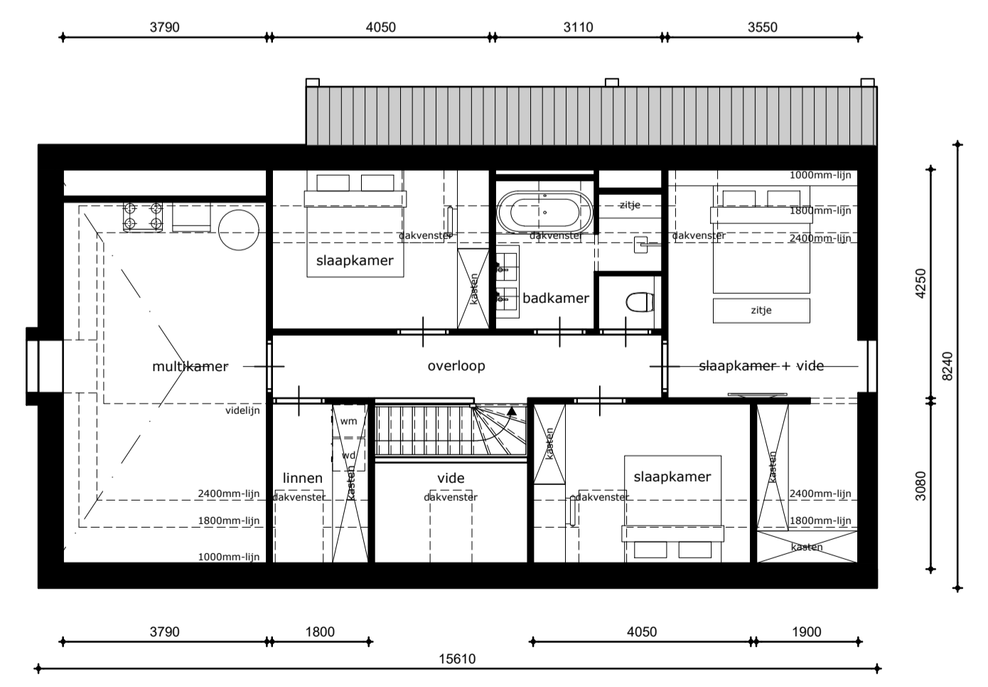
-- 1e verdieping --
