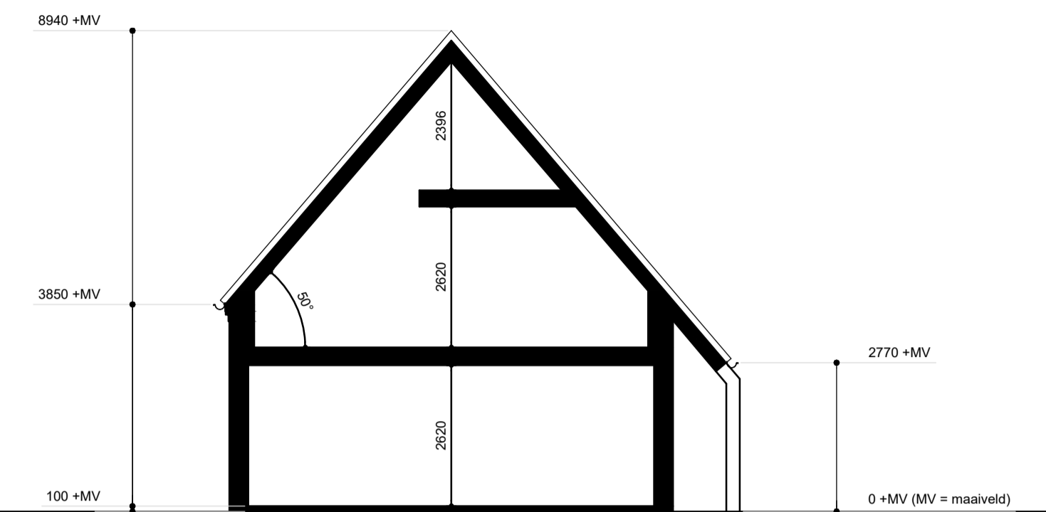
-- doorsnede 55 --
