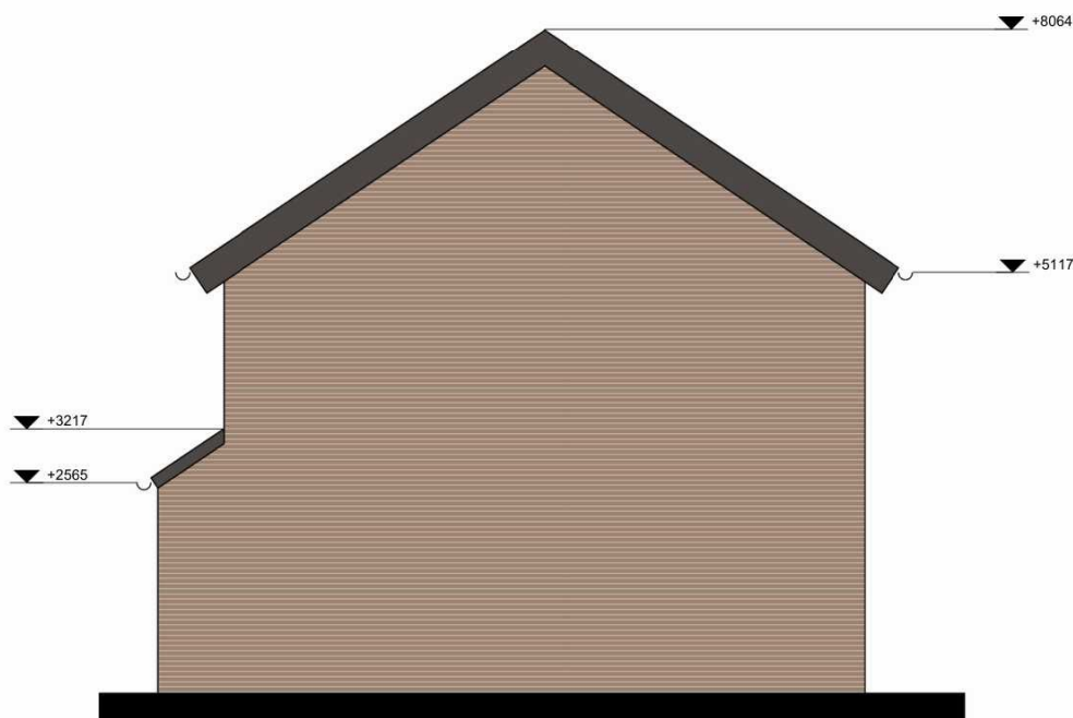
Zijgevel
