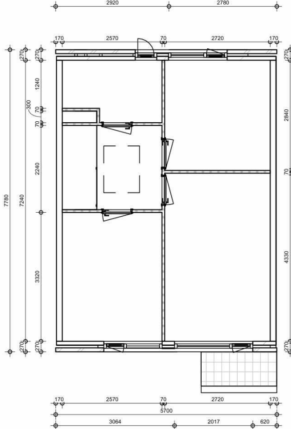
eerste verdieping
