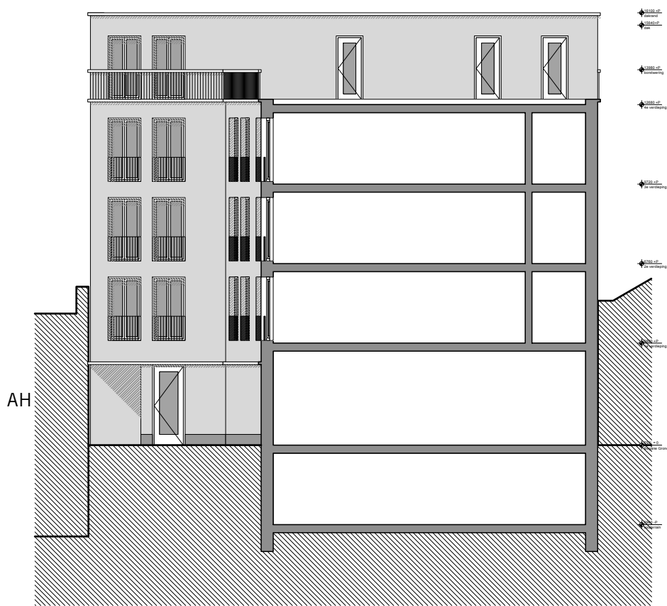
DOORSNEDE B
