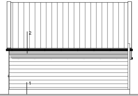
Rechtergevel bijgebouw
