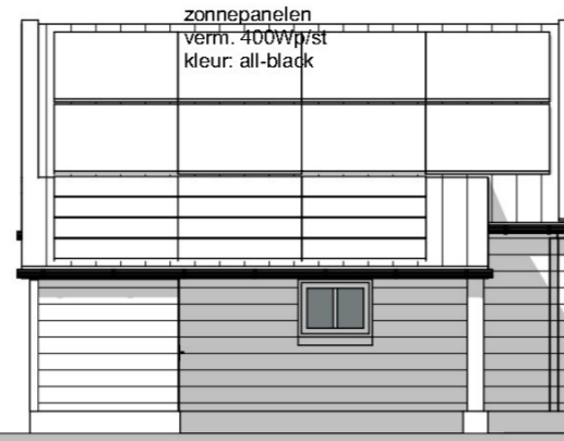
Linkergevel bijgebouw
