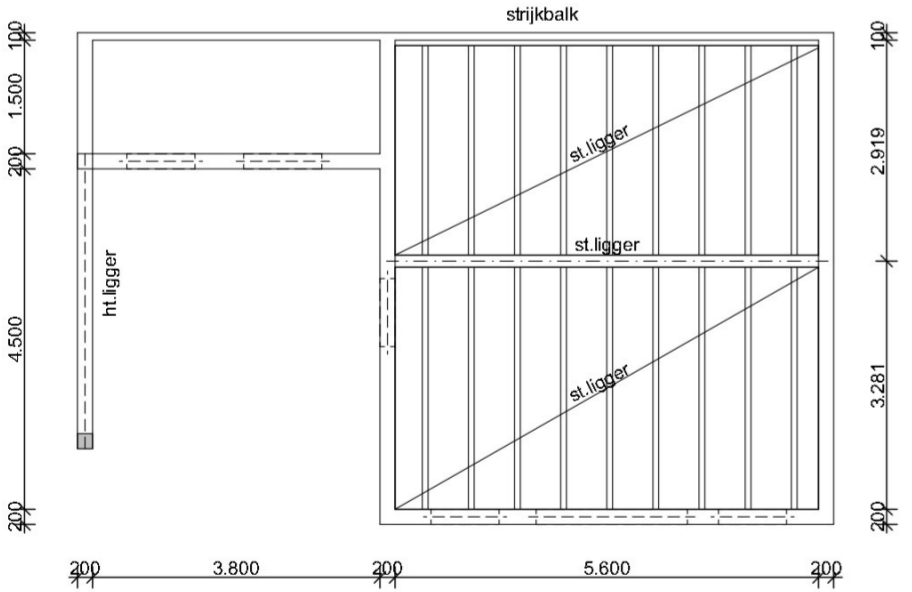
Balklagen
