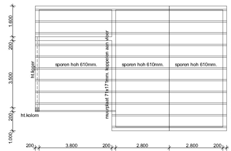
kapplan
