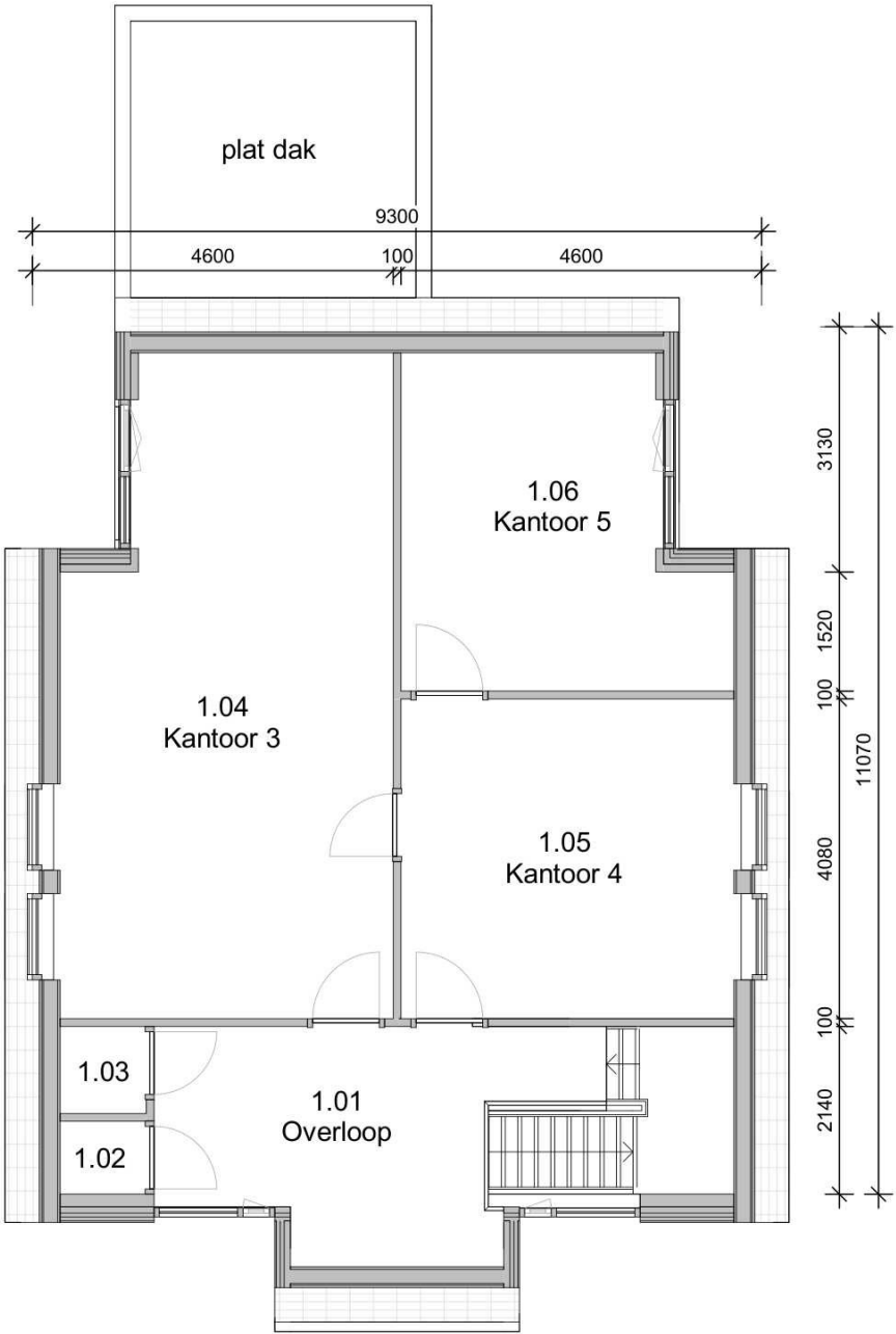
Eerste verdieping bestand
