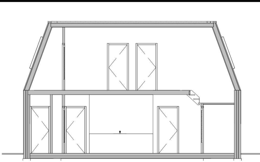
Principedoorsnede BB bestand
