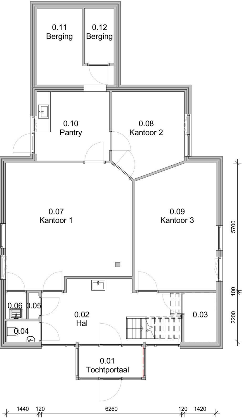
Begane grond bestand
