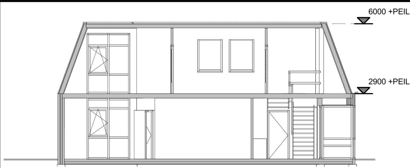
Principedoorsnede AA bestand
