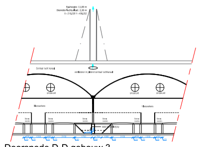
Doorsnede D-D gebouw 3
