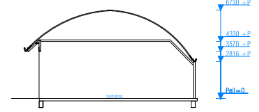
Doorsnede gebouw 9
