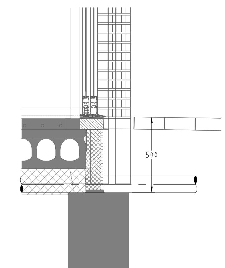
detail 4892W-VO-Z00
