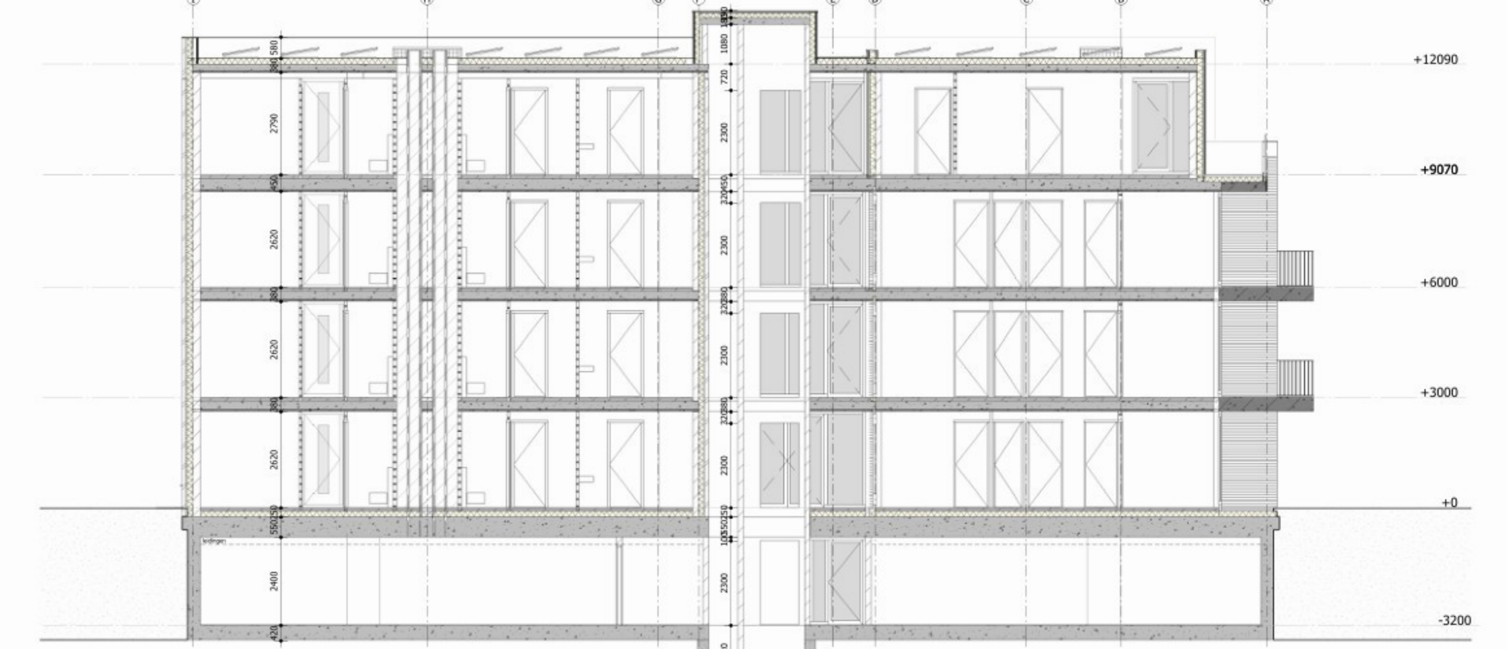
Doorsnede EE
