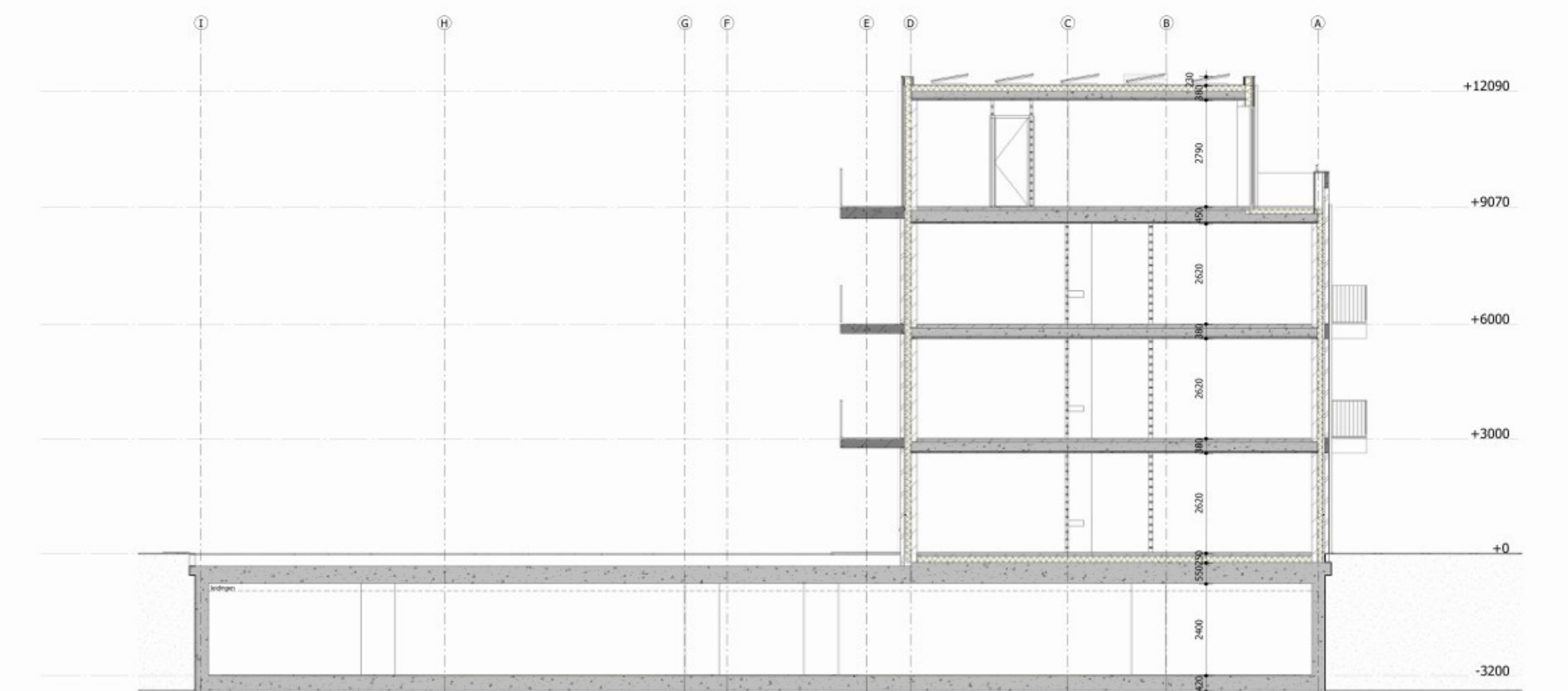
Doorsnede FF
