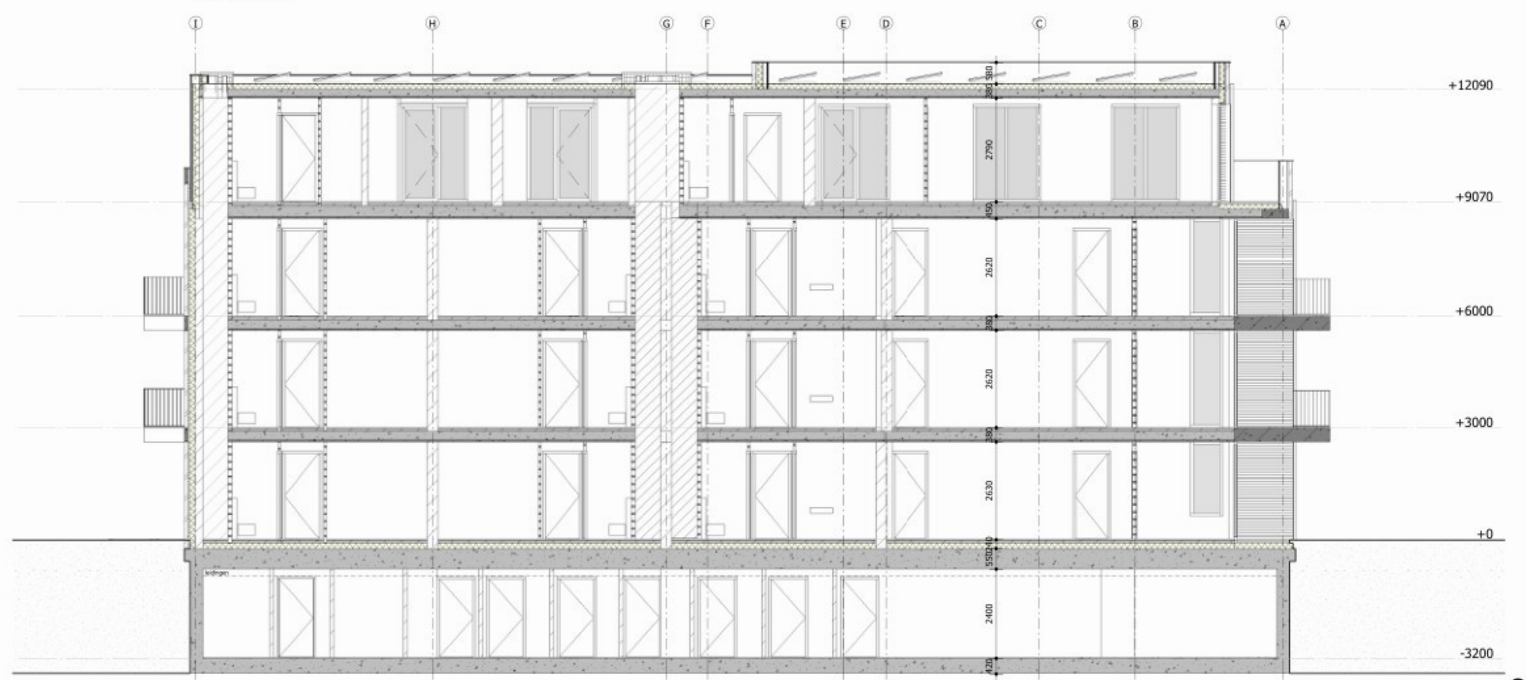
Doorsnede HH
