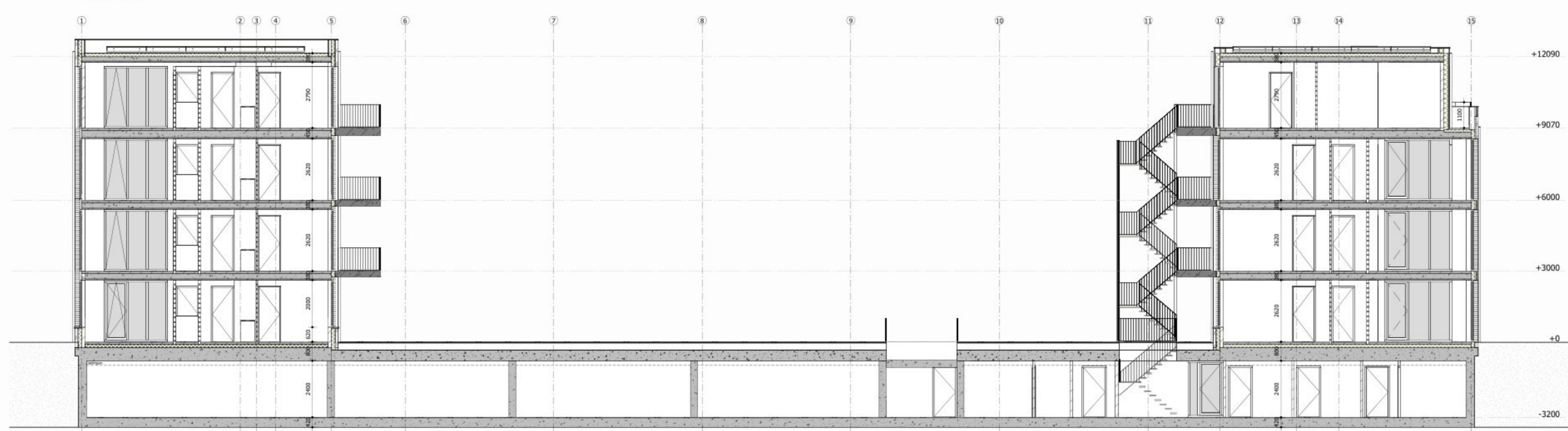
Doorsnede DD
