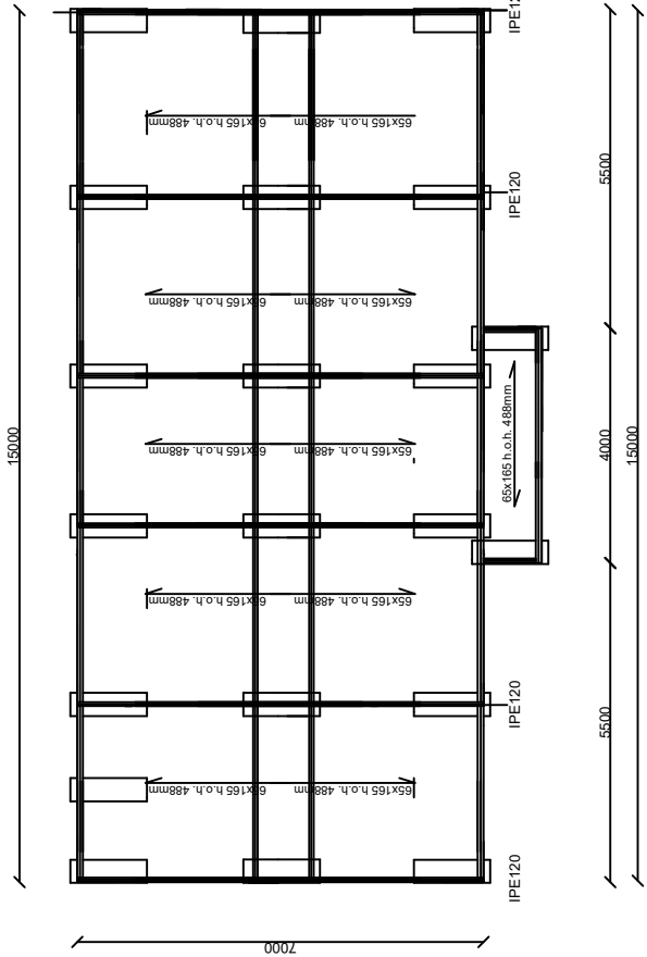
CONSTRUCTIE FUNDERINGVLOER
