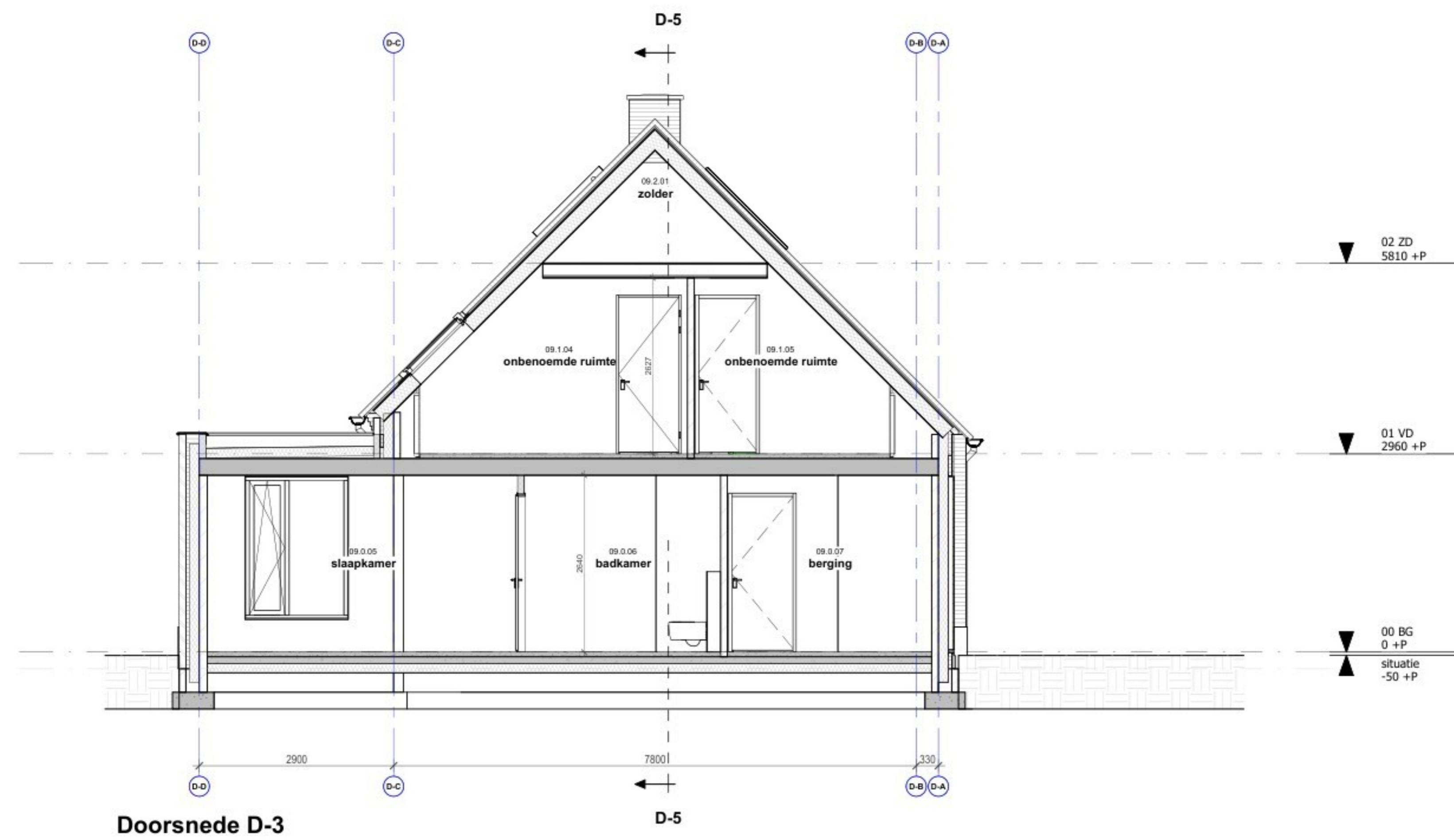
Doorsnede D-3
