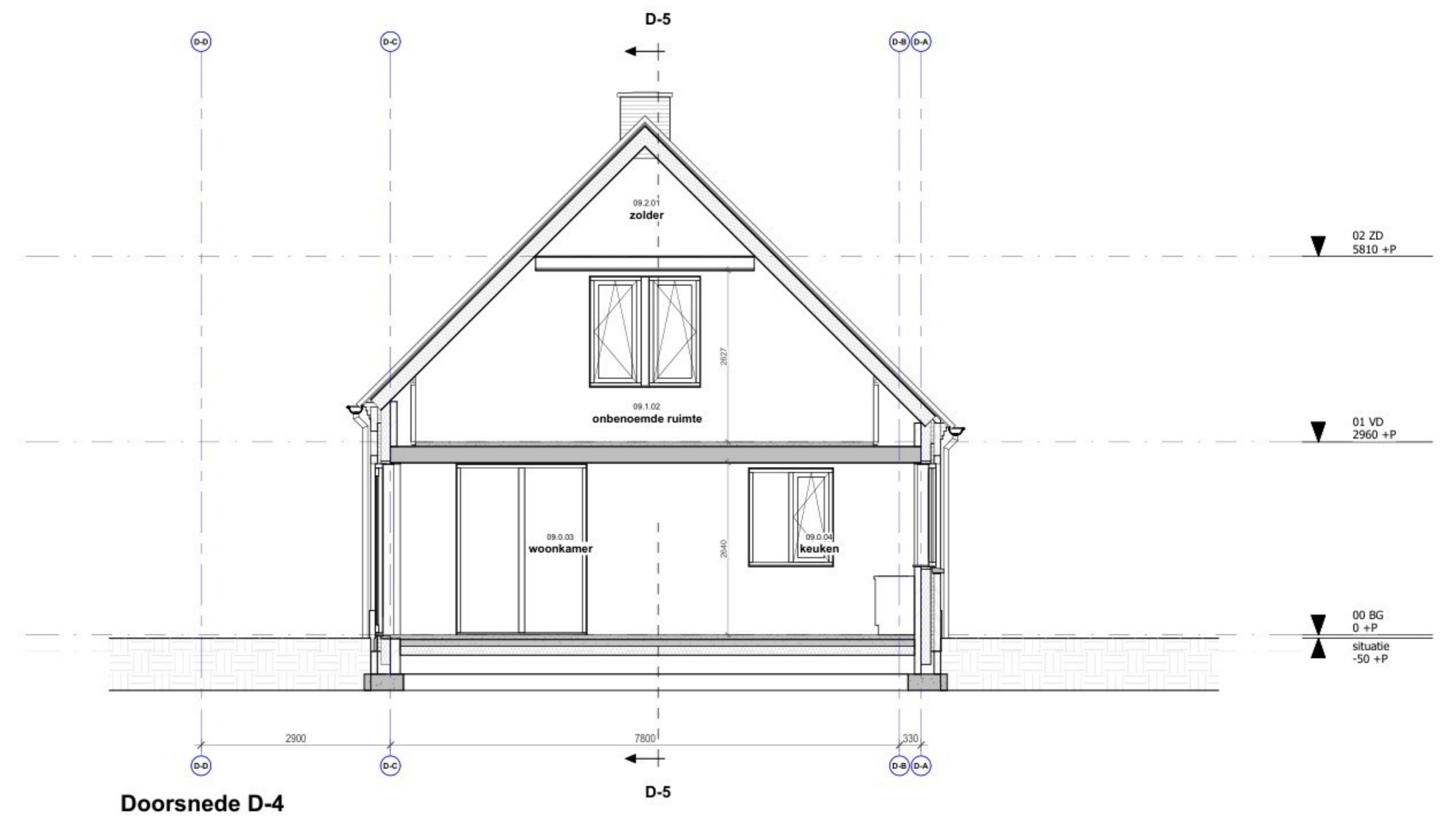
Doorsnede D-4
