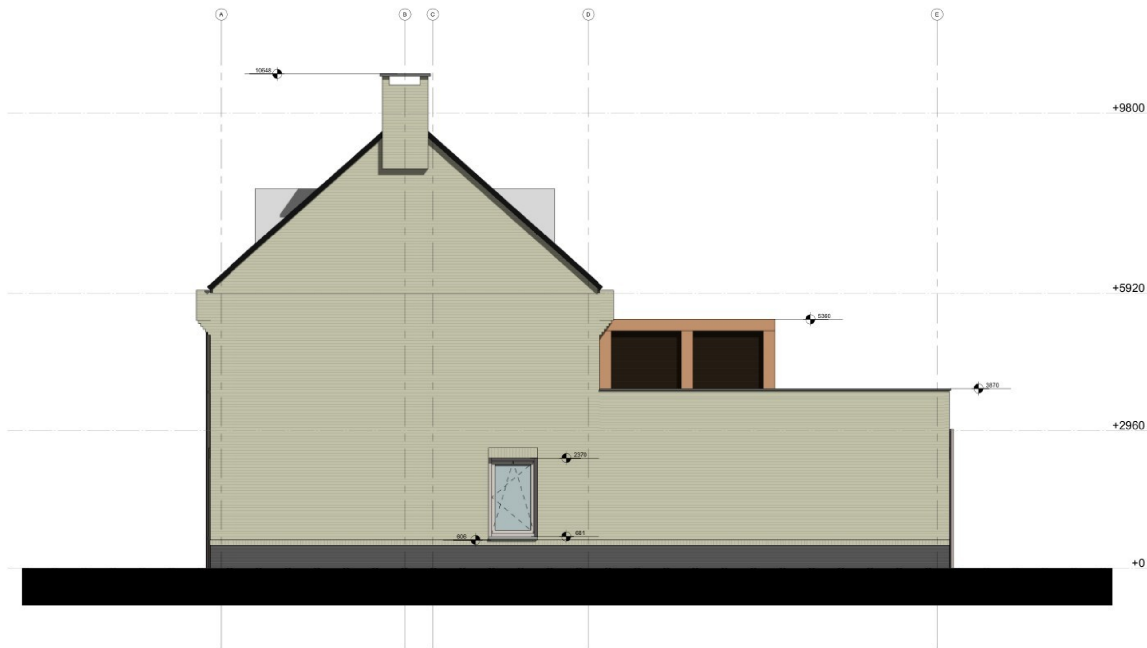
2 Rechtergevel 1 : 50
