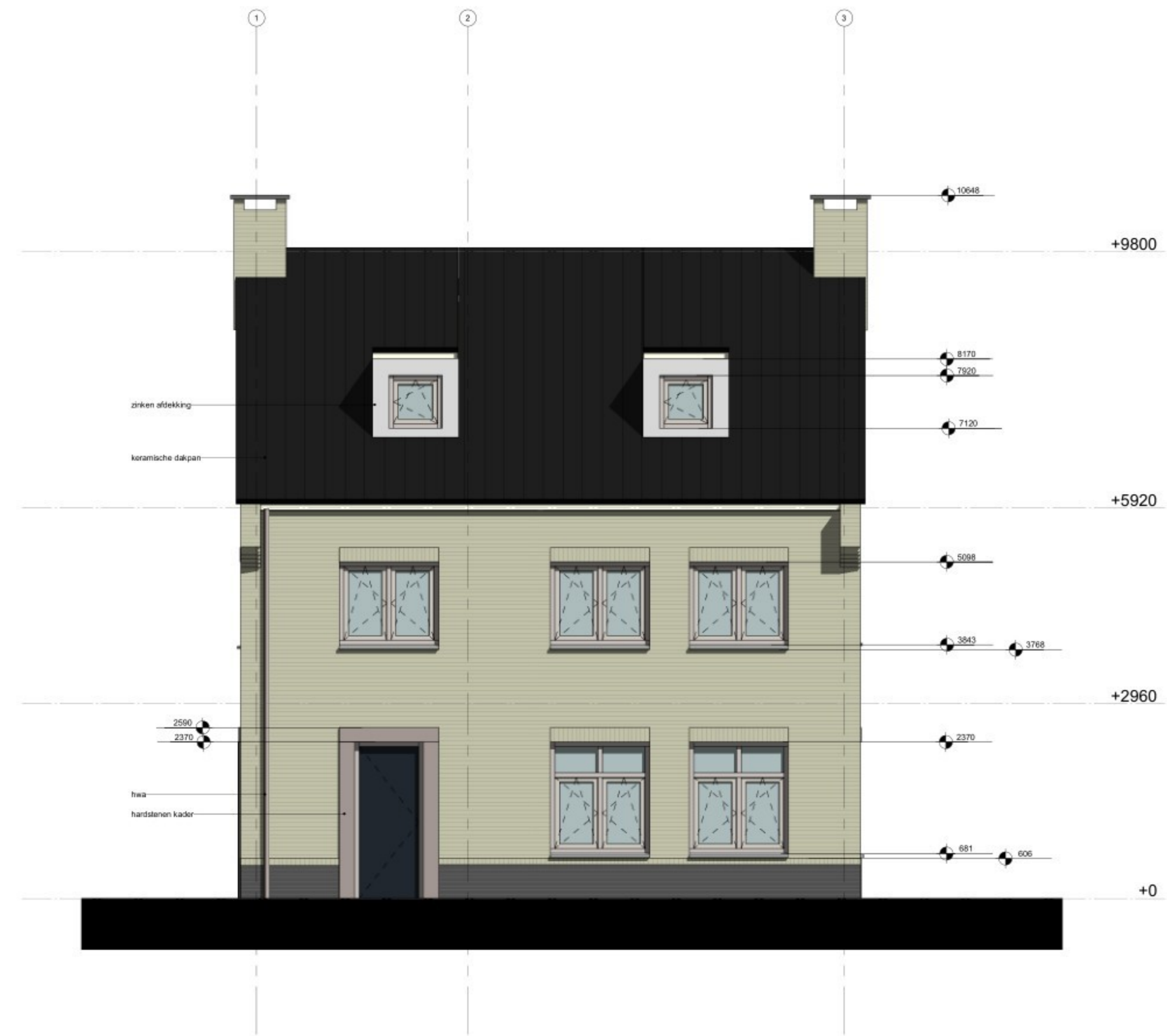
1 Voorgevel 1 : 50
