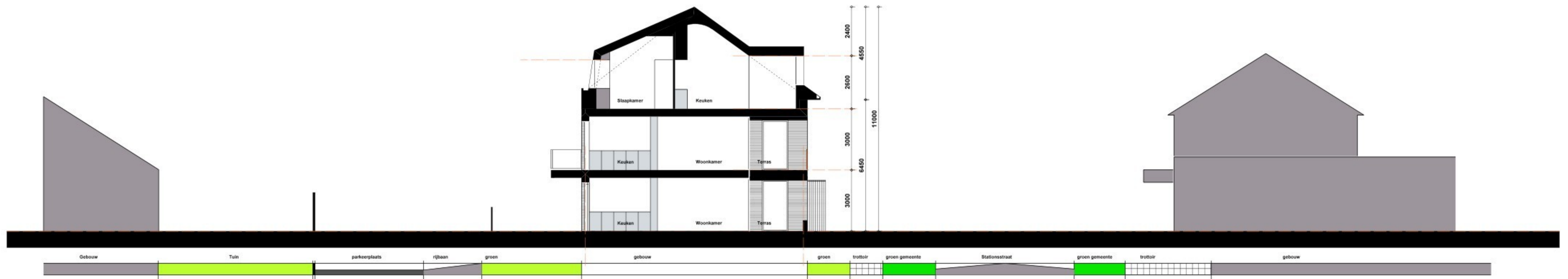
Doorsnede 04
