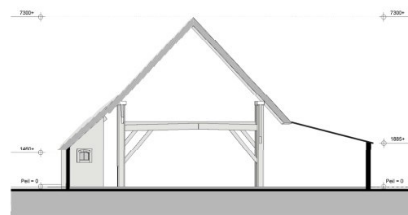
DOORSNEDE A (BESTAAND)
