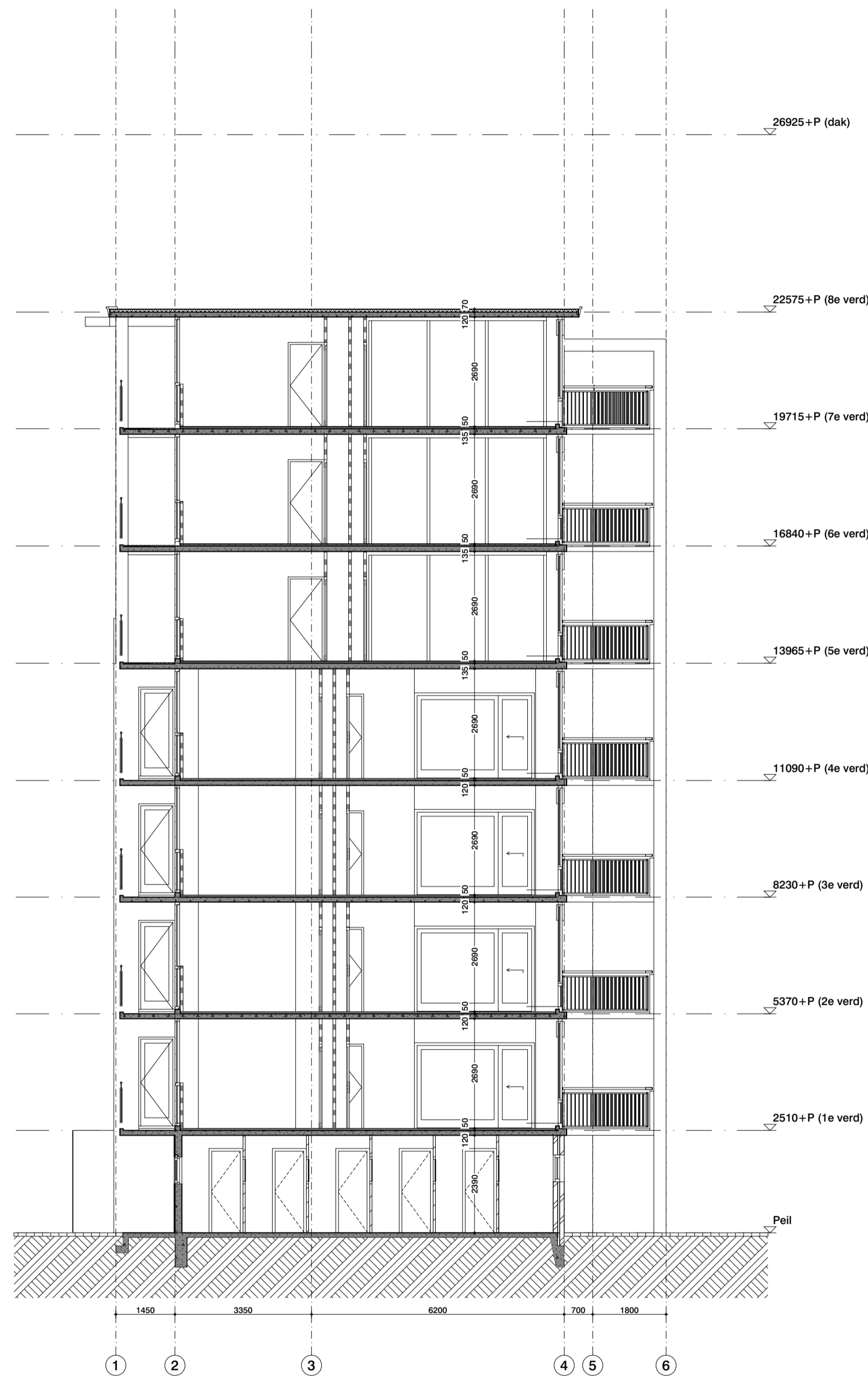
doorsnede A
