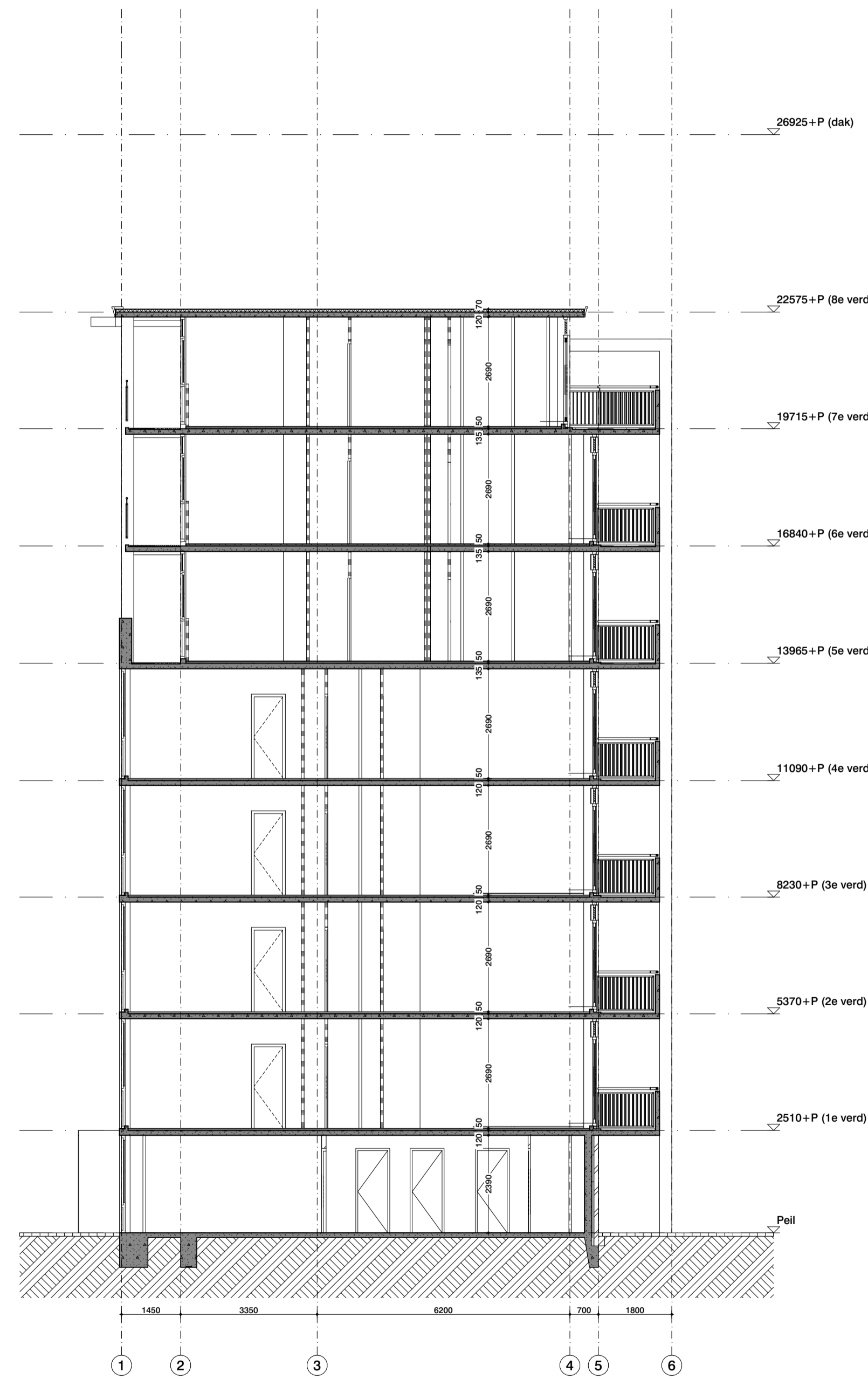
doorsnede B
