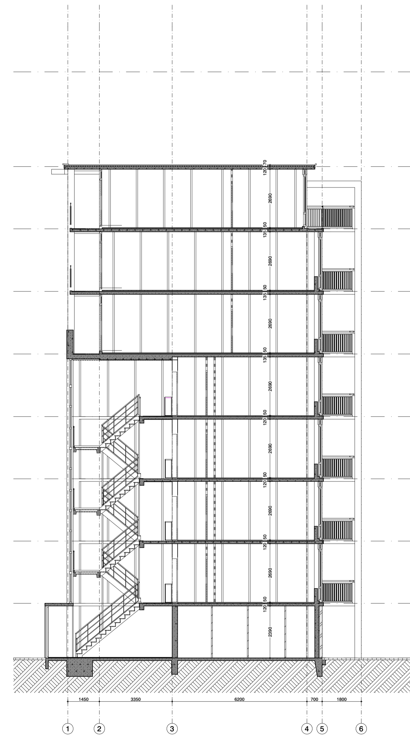
doorsnede C
