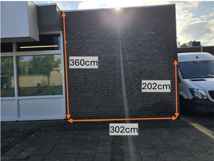
Afmetingen pakketautomaat Grond tot bovenkant muur – 360cm Hoogte pakketautomaat – 202cm Breedte pakketautomaat – 302cm
