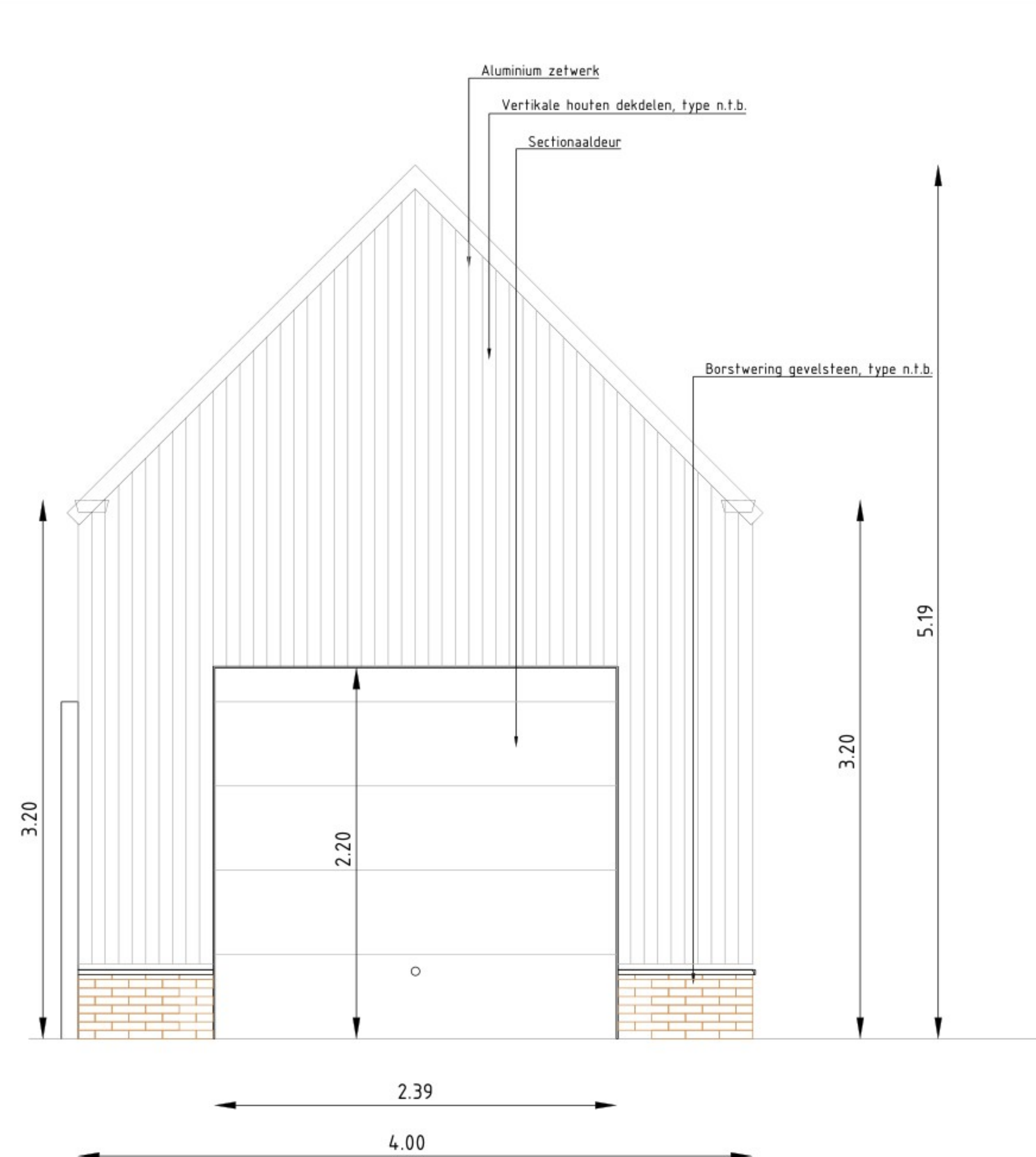
VOORAANZICHT
