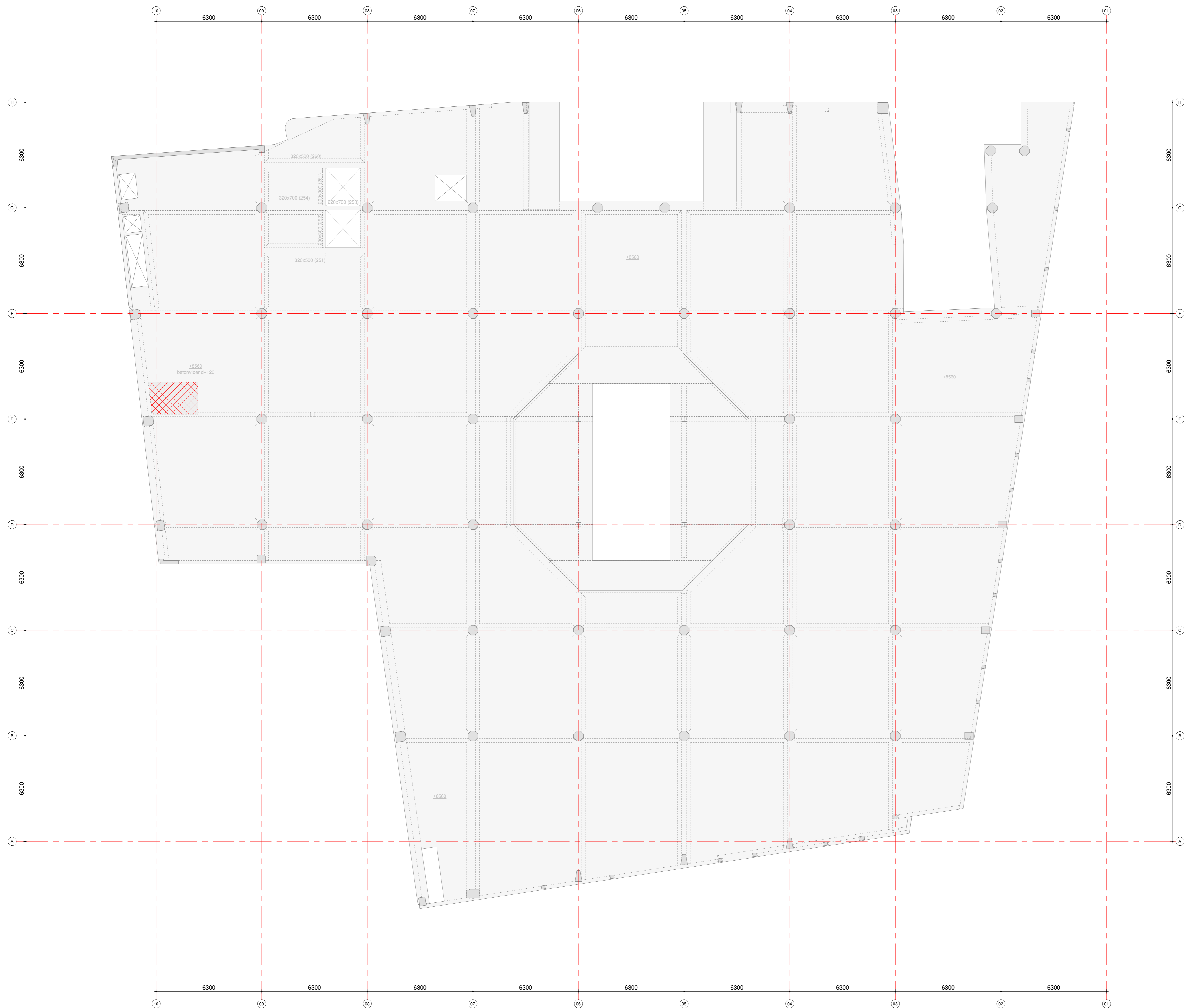
02 tweede verdieping(SL)
