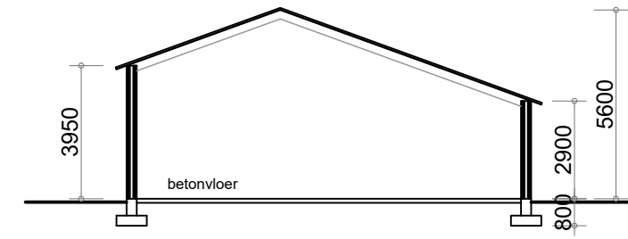
- Doorsnede C - C - gebouw 3 -
