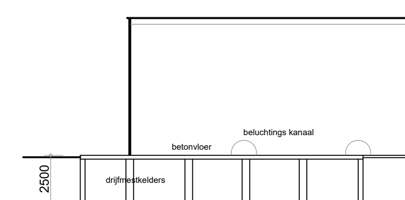
- Doorsnede G - G - gebouw 6 -
