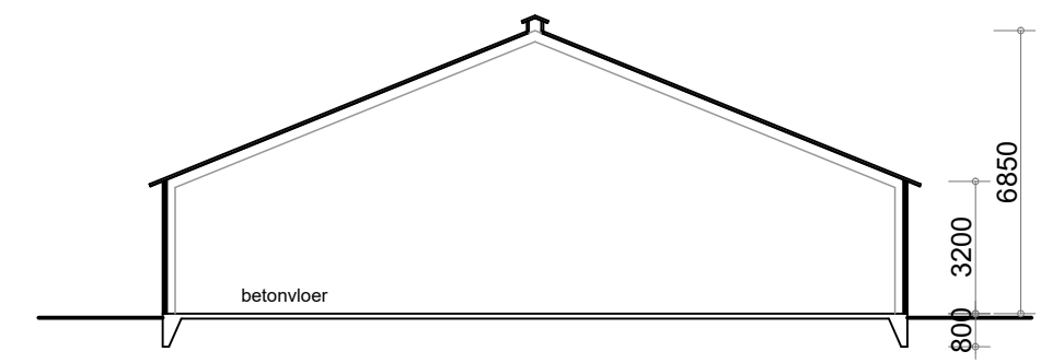
- Doorsnede A - A - gebouw 1 -
