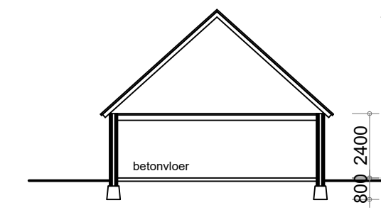
- Doorsnede E - E - gebouw 5 -
