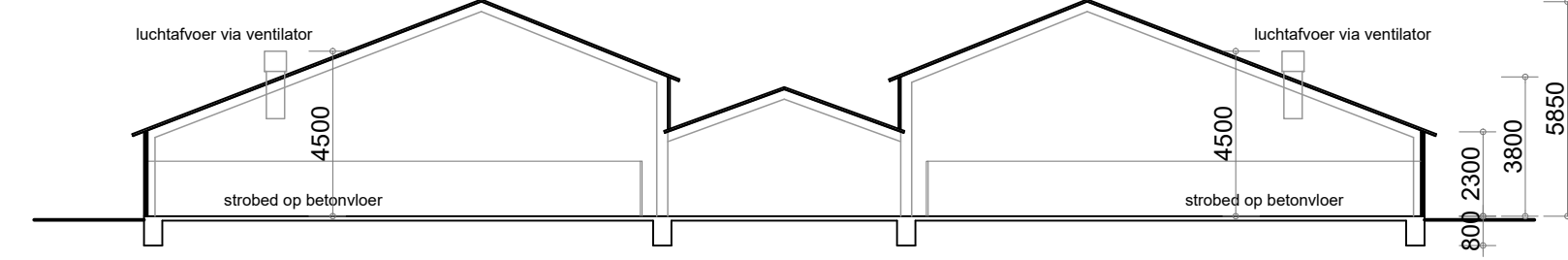
- Doorsnede D - D - gebouw 4 -
