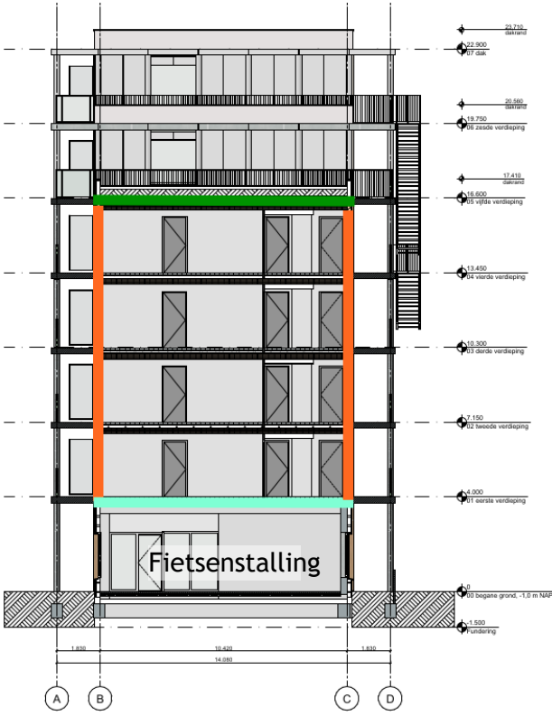
Dwarsdoorsnede F-F
