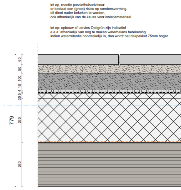
Detail opbouw vloer dakterras
