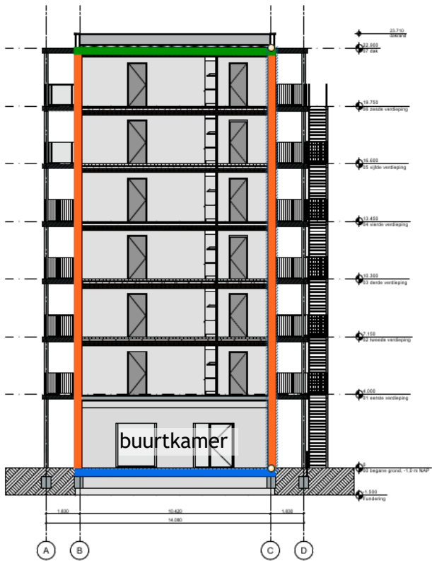
Dwarsdoorsnede A-A
