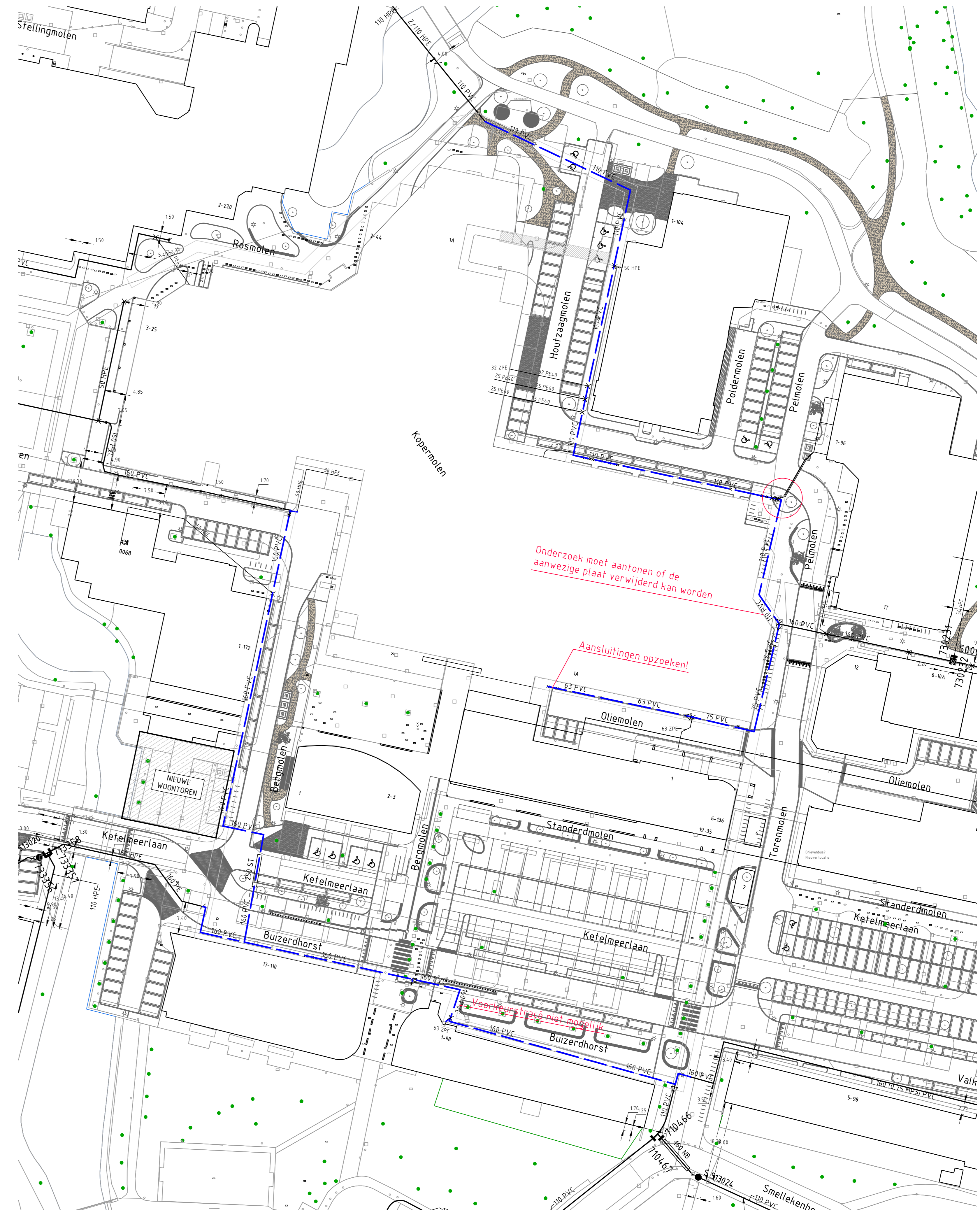
Nieuwe situatie
