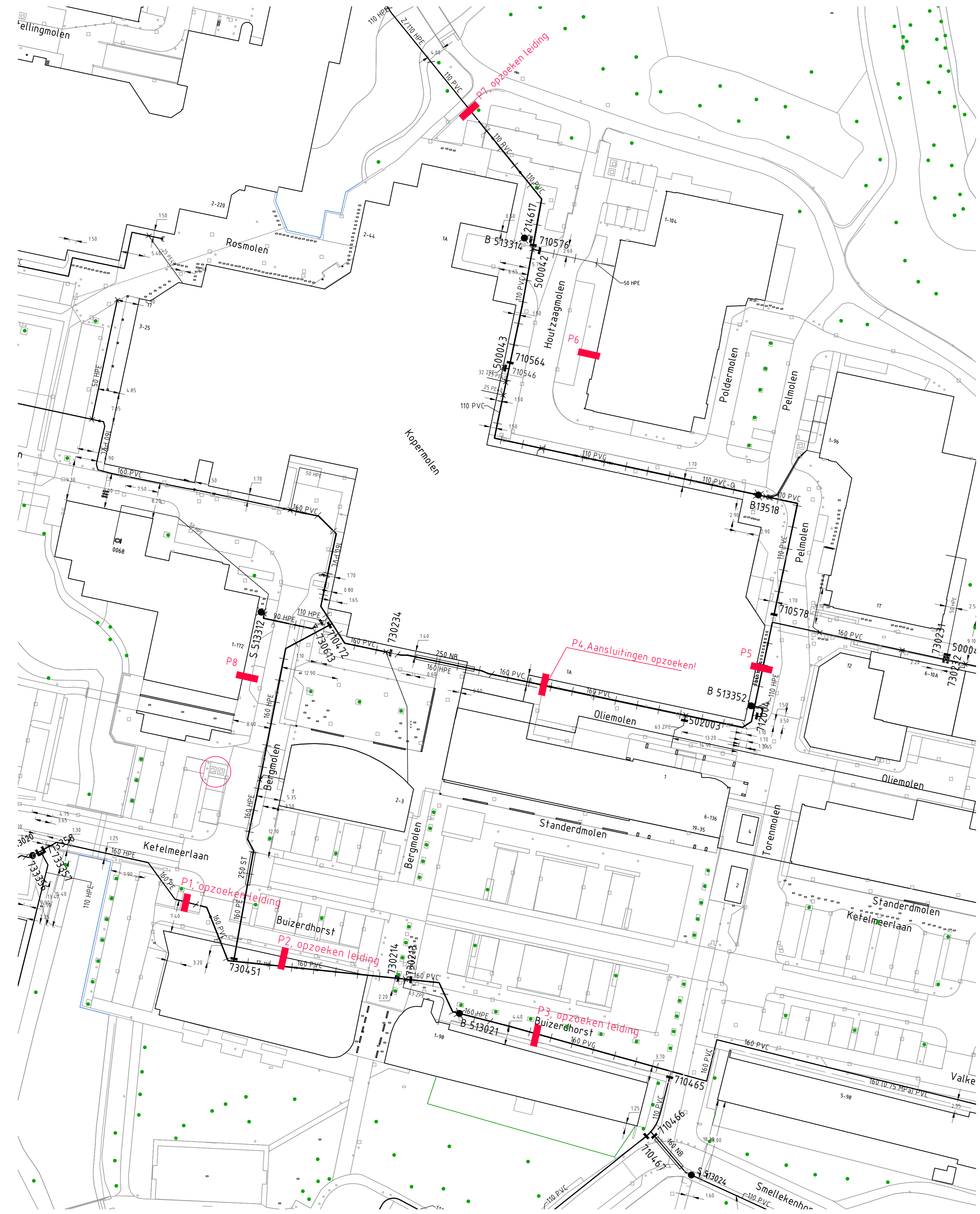
Bestaande situatie
