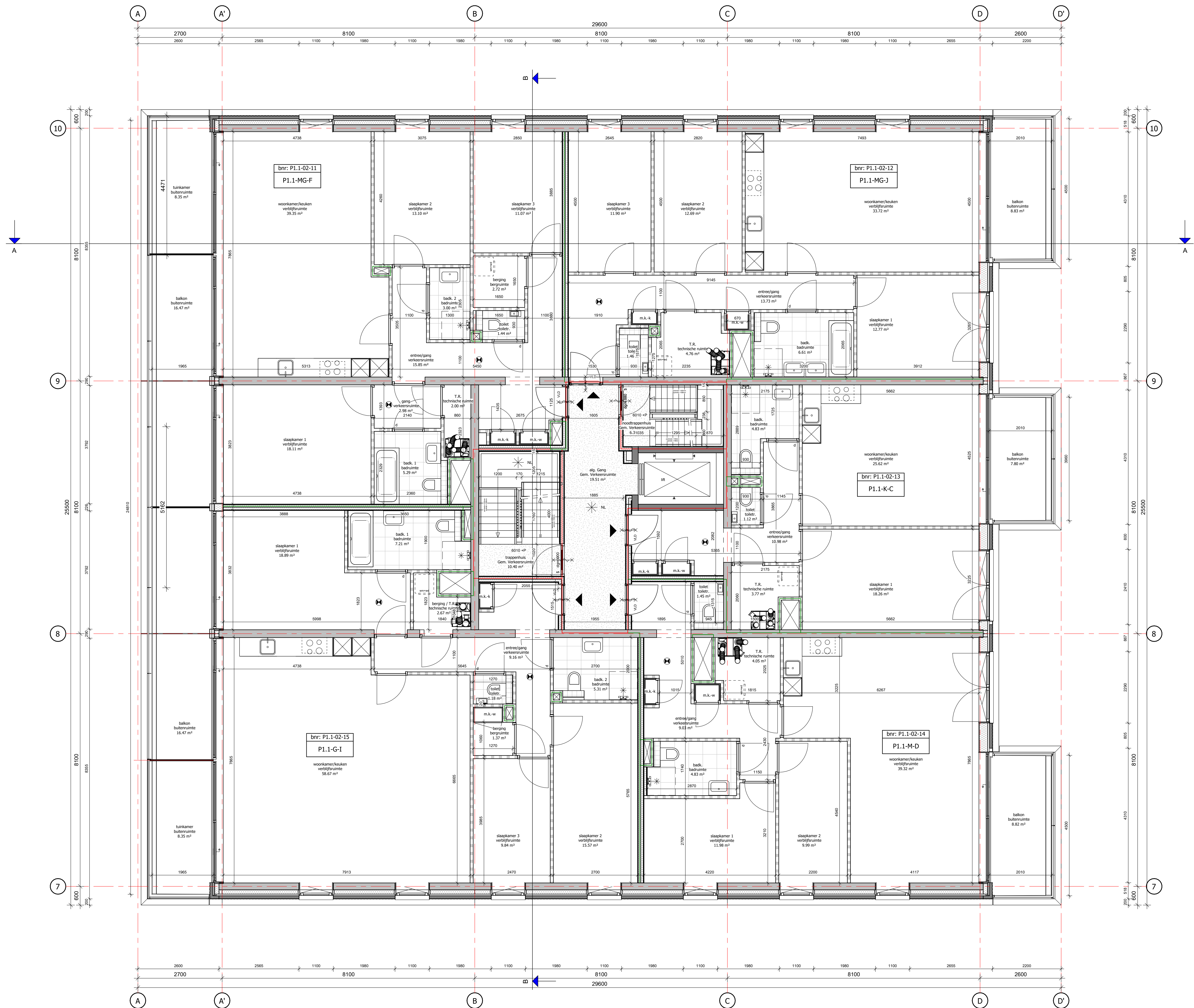
Tweede verdieping schaal 1:50
