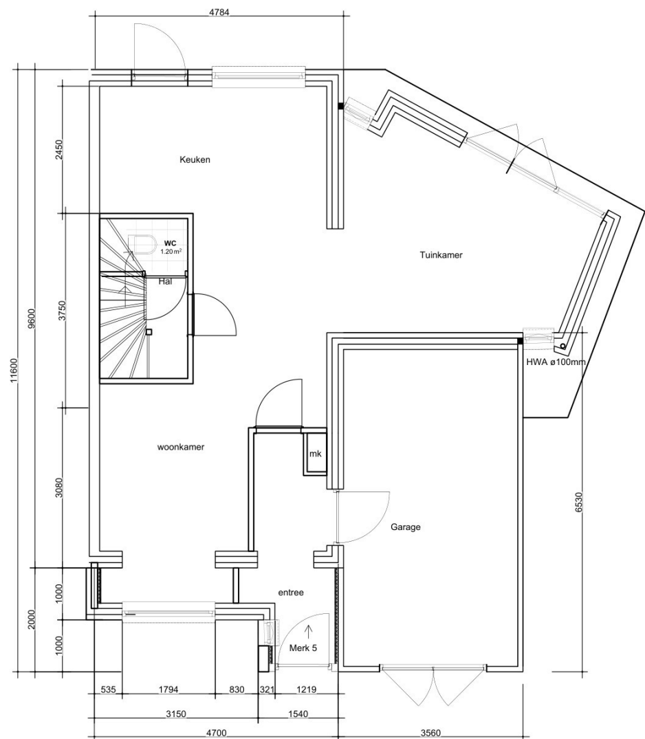
Plattegrond Nieuw
