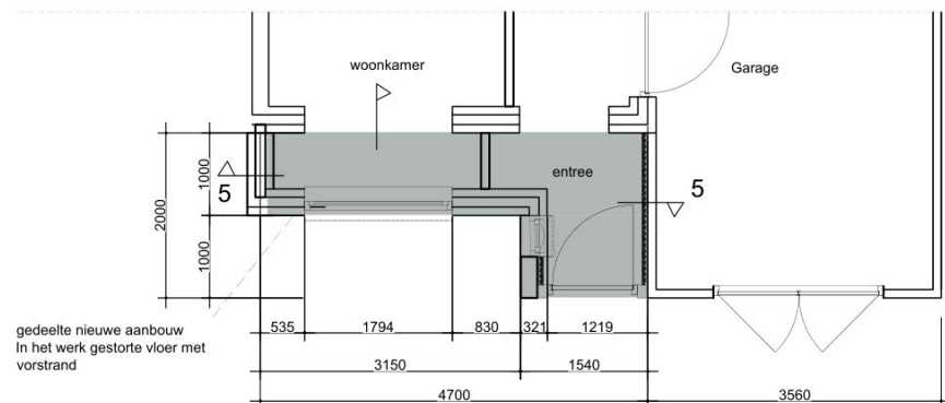
Fundering / Vloer
