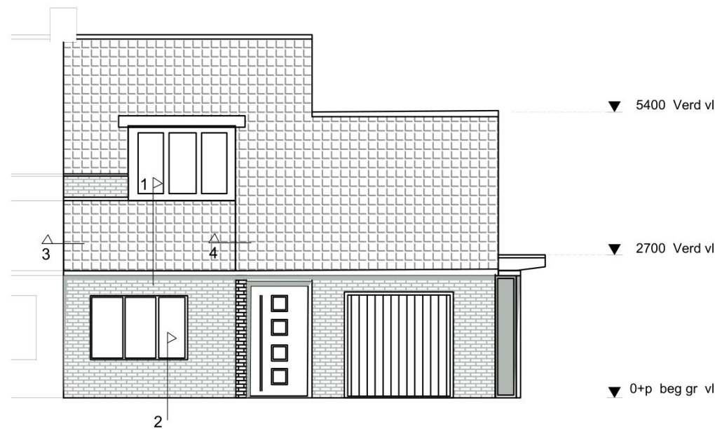
Gevelaanzicht Nieuw
